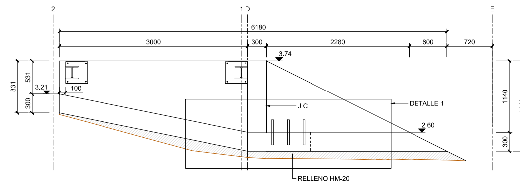
ALZADO MURO ESCALA 1:30
