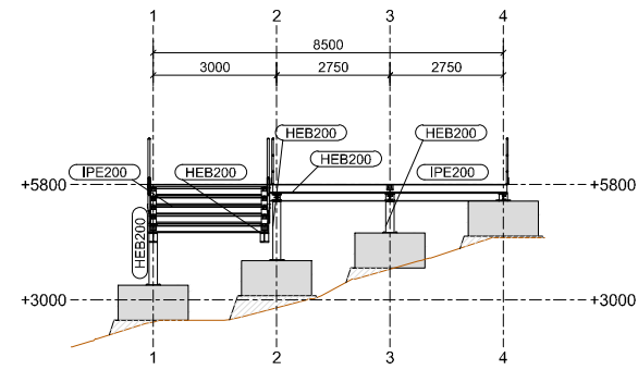
SECCIÓN EJE C ESCALA 1:100
