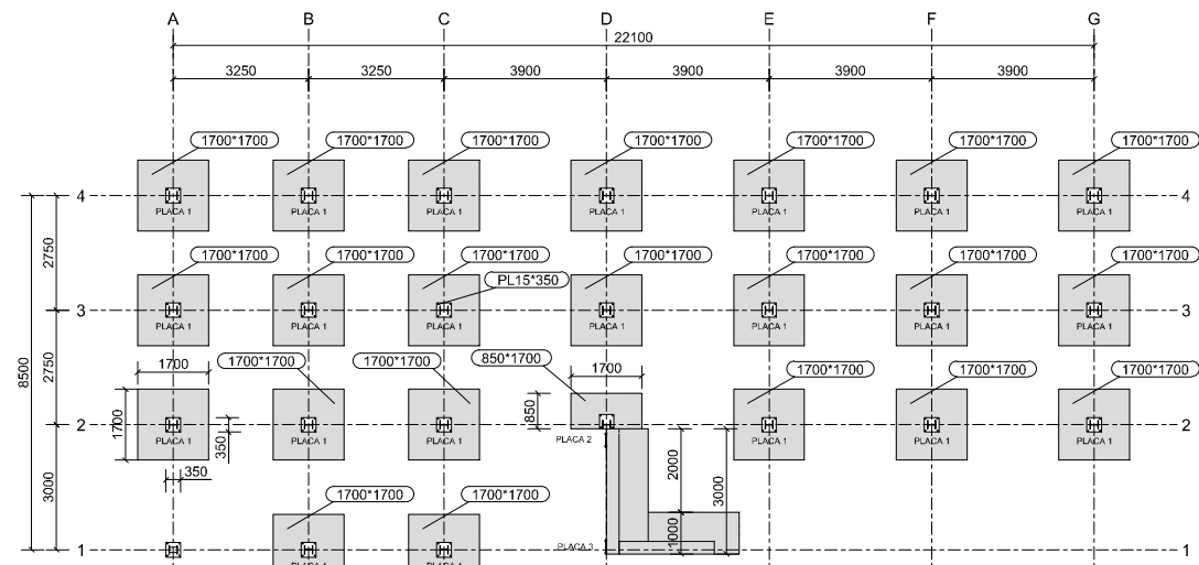
PLANTA +5394 ESCALA 1:100
