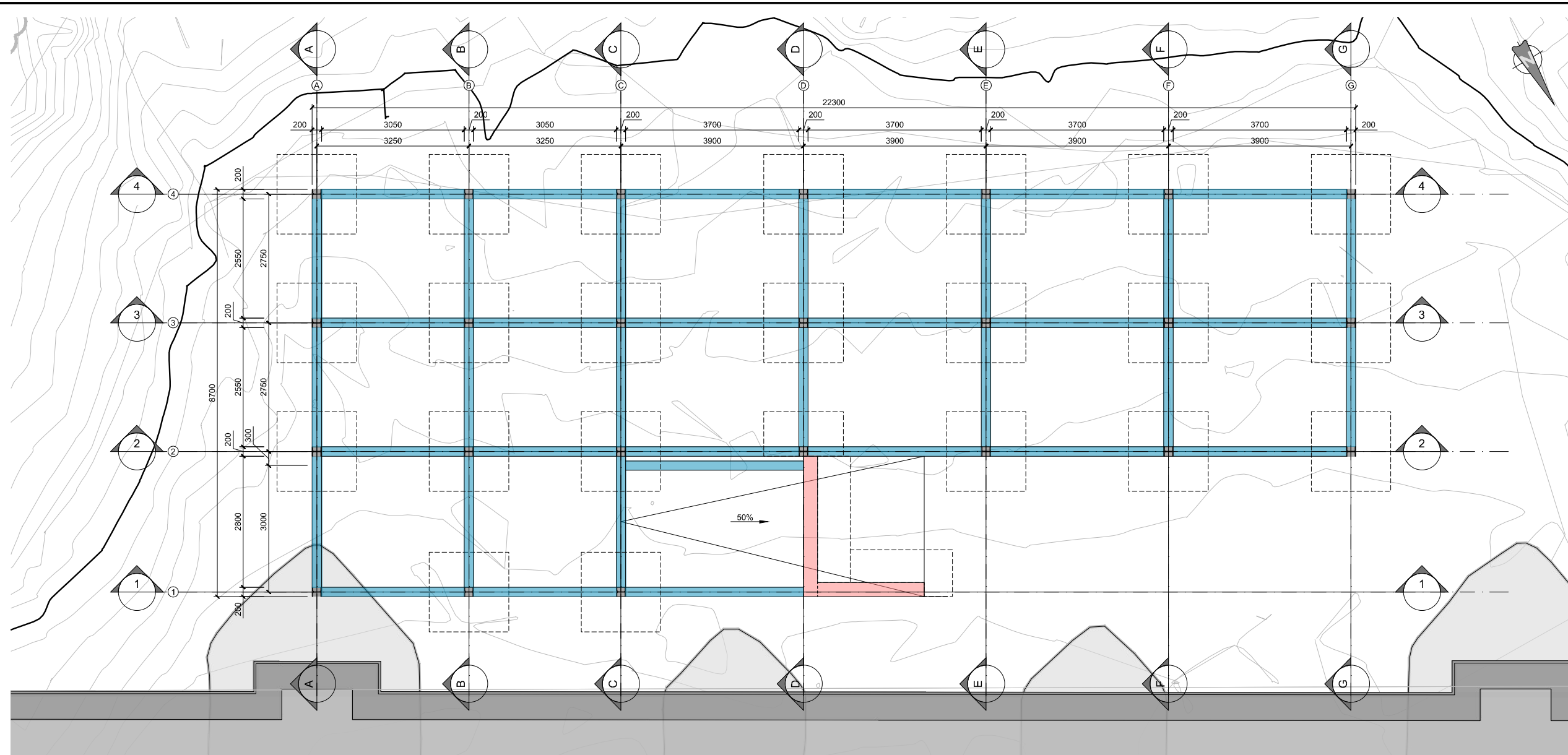
PLANTA ESCALA 1:50
