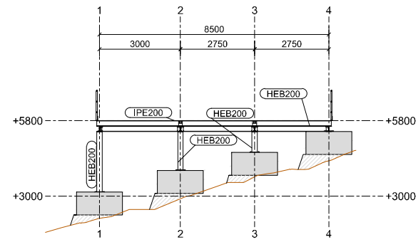
SECCIÓN EJE B ESCALA 1:100
