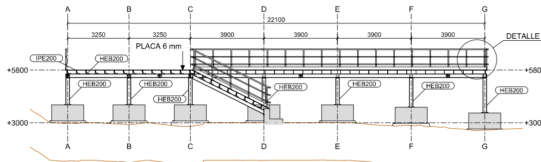
SECCIÓN EJE 2 ESCALA 1:100
