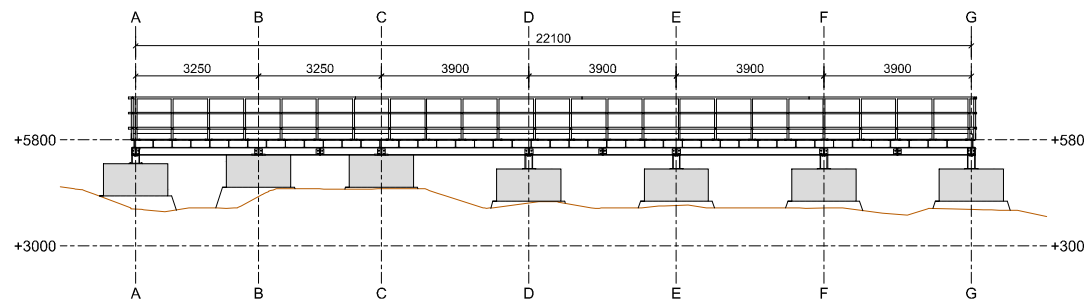
SECCIÓN EJE 4 ESCALA 1:100
