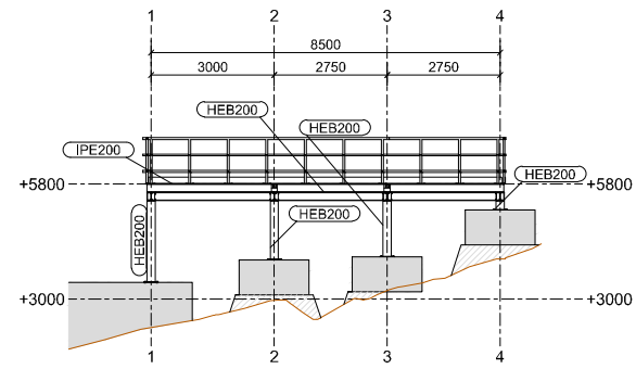
SECCIÓN EJE A ESCALA 1:100
