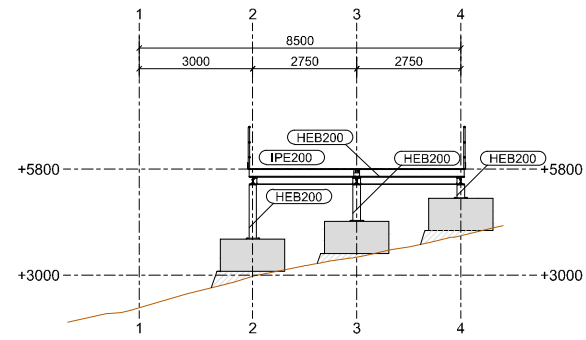
SECCIÓN EJE E ESCALA 1:100
