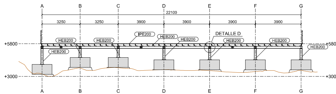
SECCIÓN EJE 3 ESCALA 1:100
