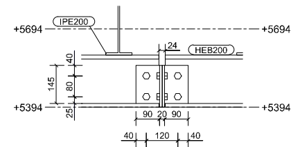
DETALLE C ESCALA 1:10
