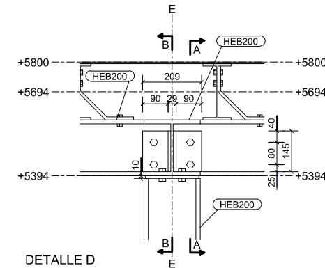
DETALLE D ESCALA 1:10
