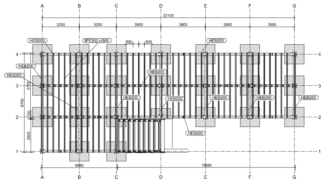
PLANTA +5694 ESCALA 1:100
