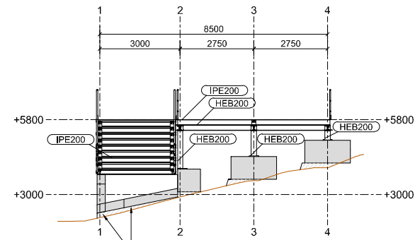
SECCIÓN EJE D ESCALA 1:100
