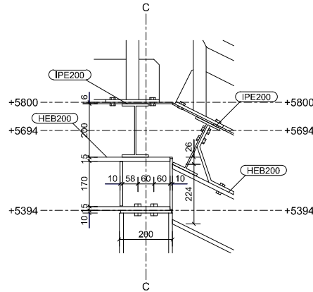
DETALLE B ESCALA 1:10
