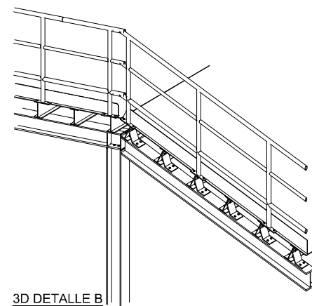
3D DETALLE B SIN ESCALA
