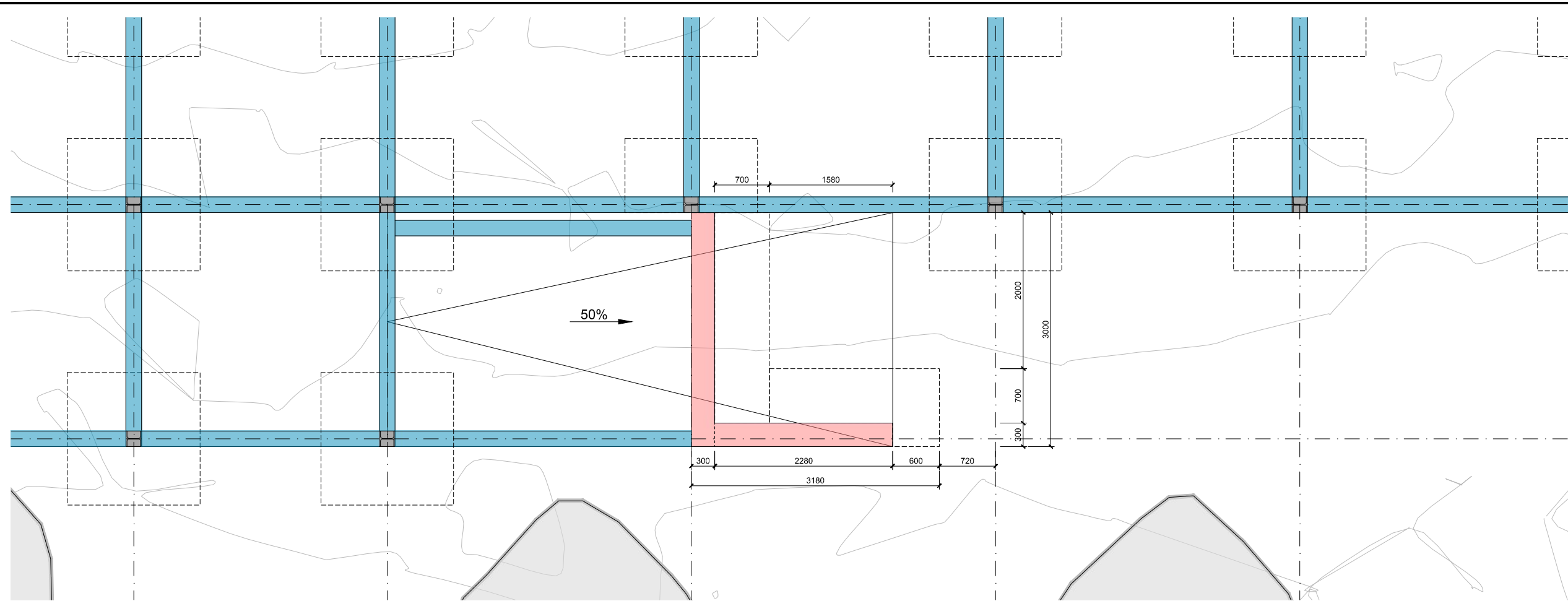
PLANTA MURO ESCALA 1:30
