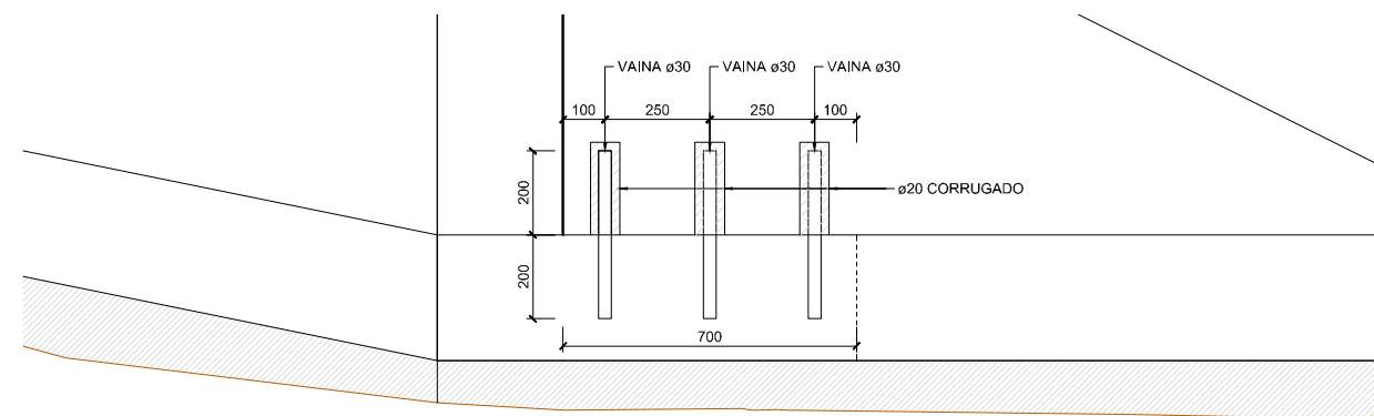
DETALLE 1 ESCALA 1:10
