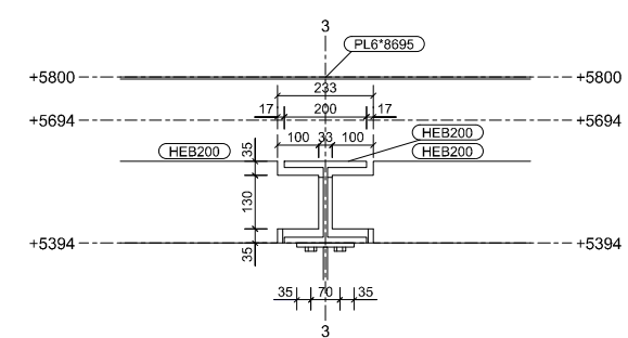
SECCIÓN B-B ESCALA 1:10
