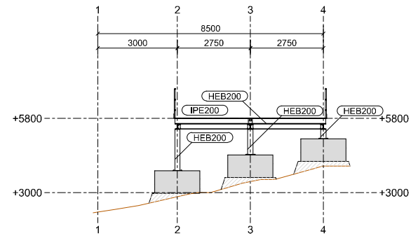
SECCIÓN EJE F ESCALA 1:100
