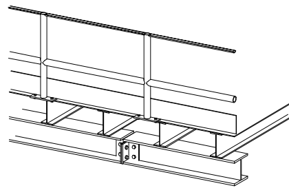
3D DETALLE C SIN ESCALA
