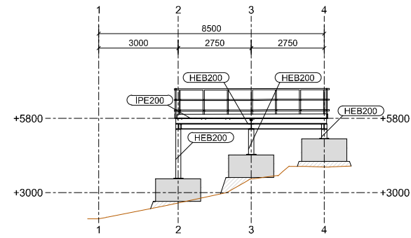
SECCIÓN EJE G ESCALA 1:100
