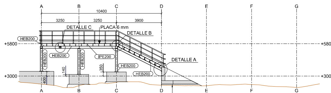
SECCIÓN EJE 1 ESCALA 1:100
