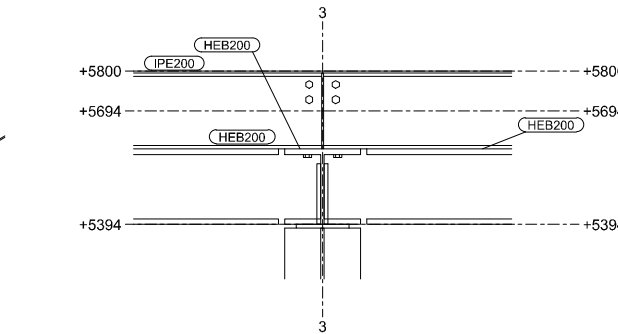
SECCIÓN A-A ESCALA 1:10
