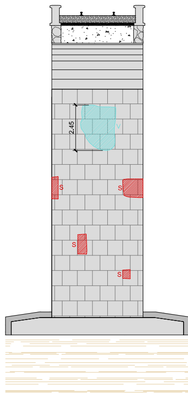
SECCIÓN E1-BERMEO ESCALA 1:100
