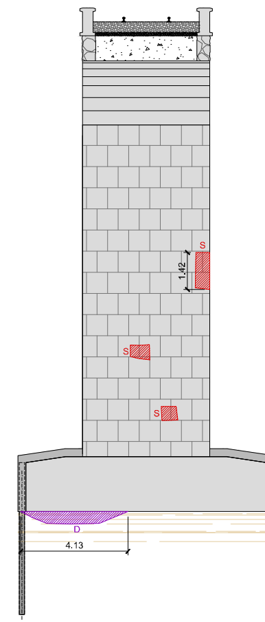
SECCIÓN P6-MUNDAKA ESCALA 1:100
