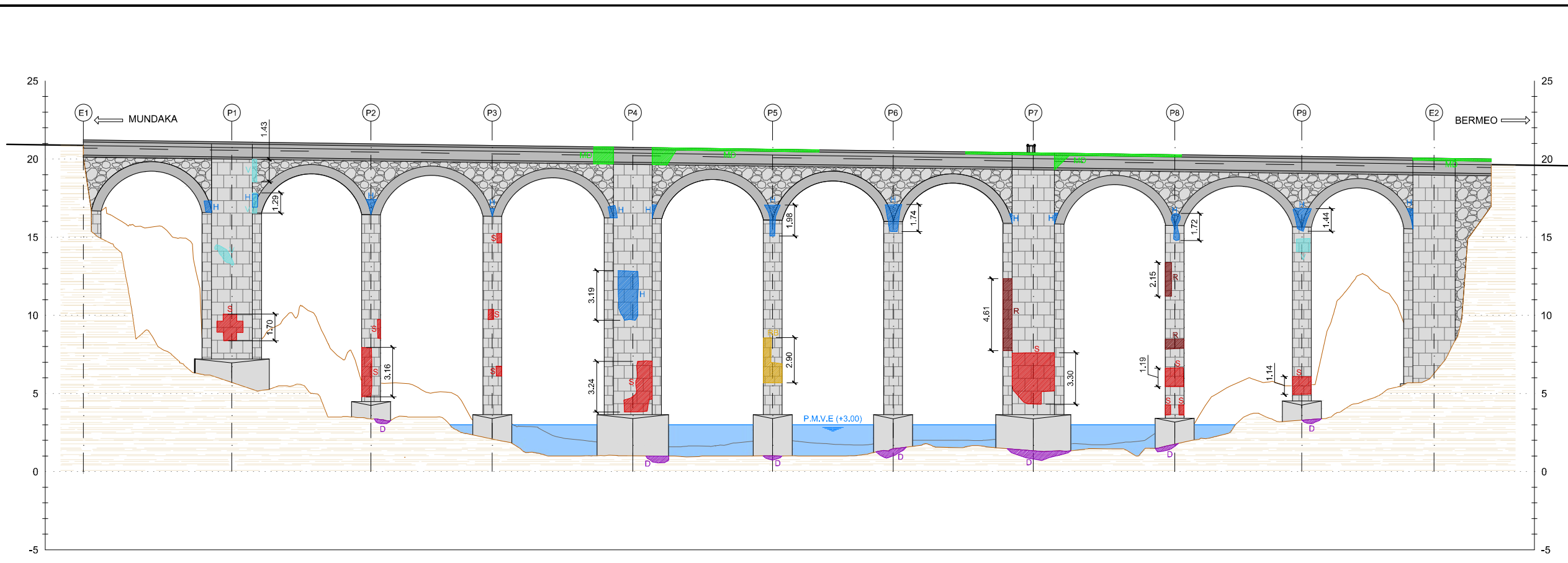
MAPA DE DAÑOS-ALZADO LADO MAR ESCALA 1:150
