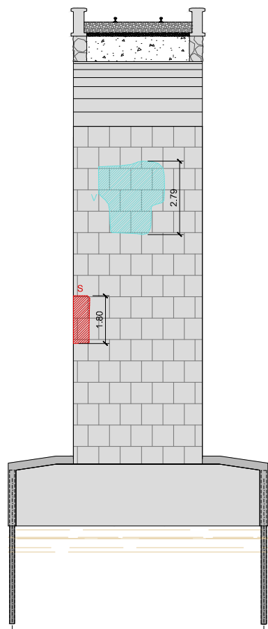
SECCIÓN P5-MUNDAKA ESCALA 1:100
