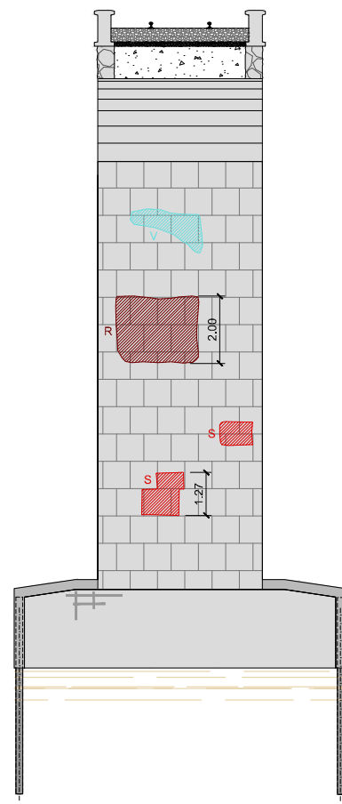
SECCIÓN P5-BERMEO ESCALA 1:100
