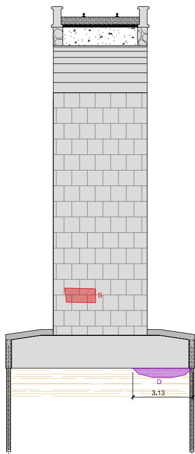
SECCIÓN P6-BERMEO ESCALA 1:100
