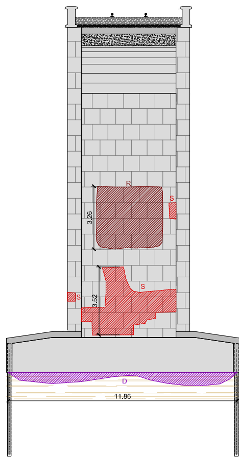
SECCIÓN P7-MUNDAKA ESCALA 1:100
