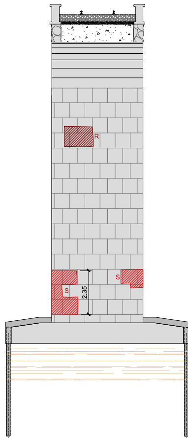
SECCIÓN P8-BERMEO ESCALA 1:100
