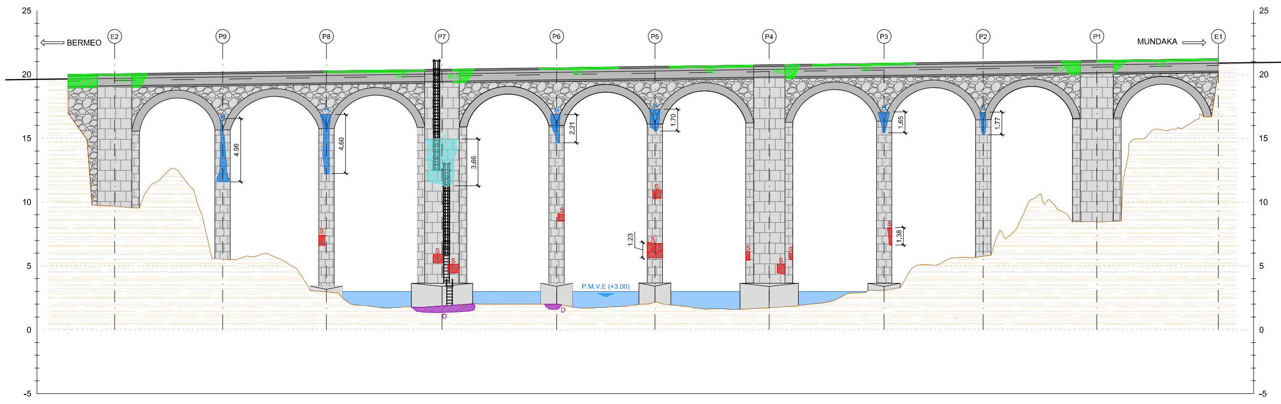
MAPA DE DAÑOS-ALZADO LADO TIERRA ESCALA 1:150
