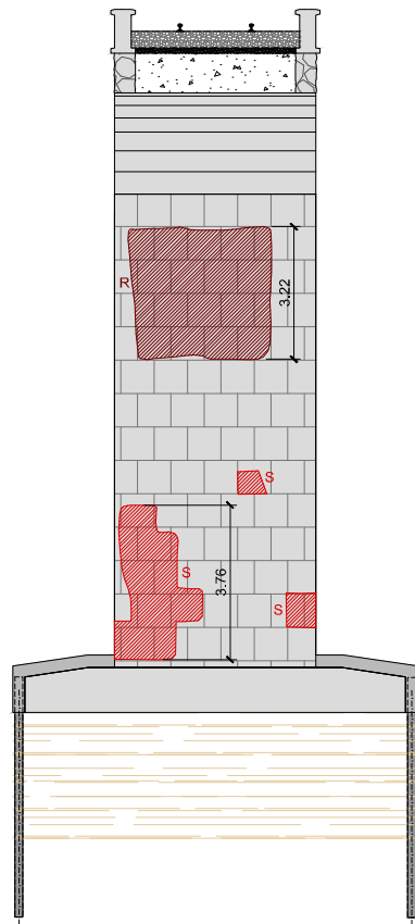
SECCIÓN P9-MUNDAKA ESCALA 1:100
