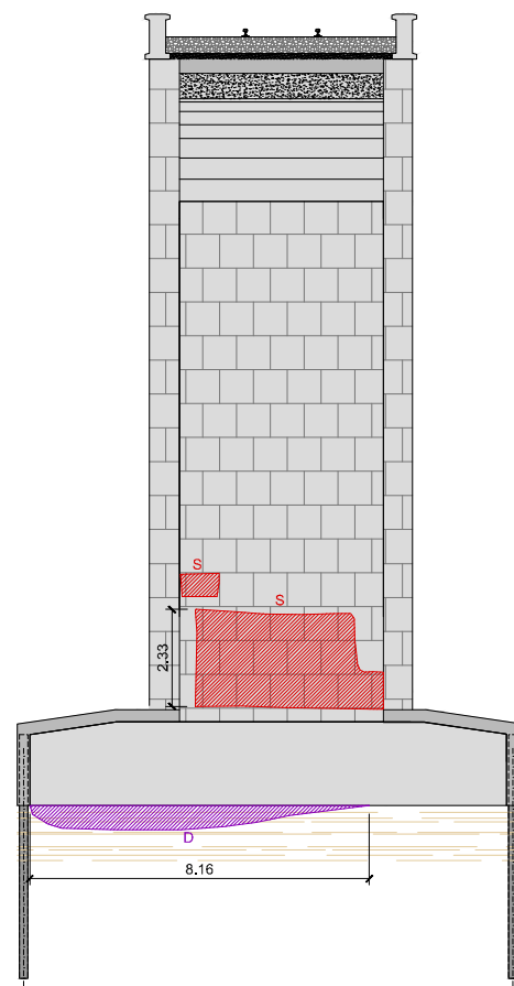
SECCIÓN P7-BERMEO ESCALA 1:100
