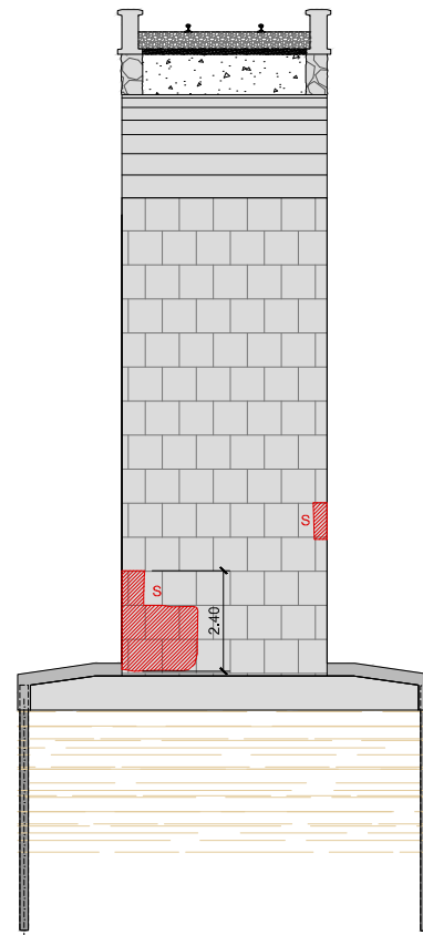
SECCIÓN P9-BERMEO ESCALA 1:100
