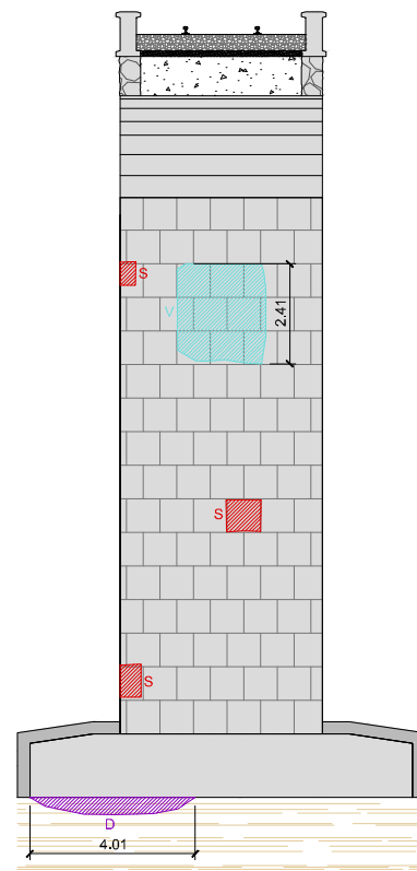
SECCIÓN P1-BERMEO ESCALA 1:100
