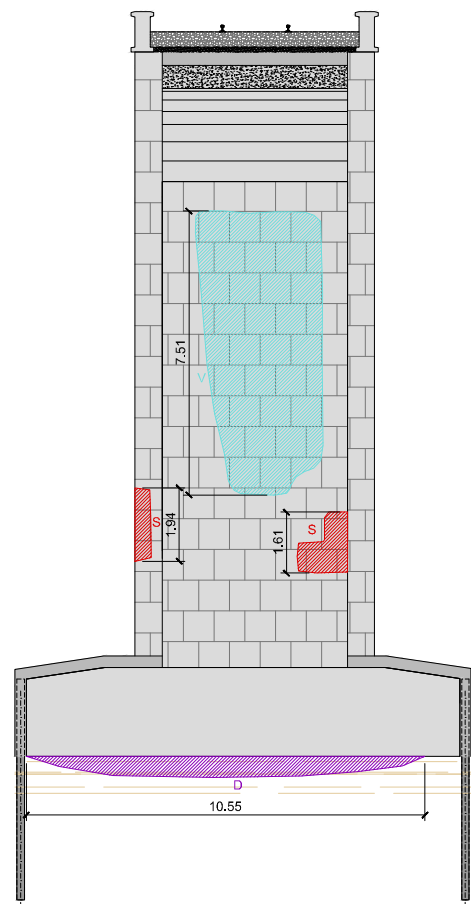
SECCIÓN P4-BERMEO ESCALA 1:100
