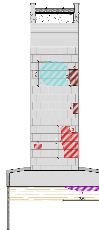
SECCIÓN P8-MUNDAKA ESCALA 1:100
