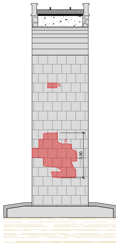
SECCIÓN P1-MUNDAKA ESCALA 1:100
