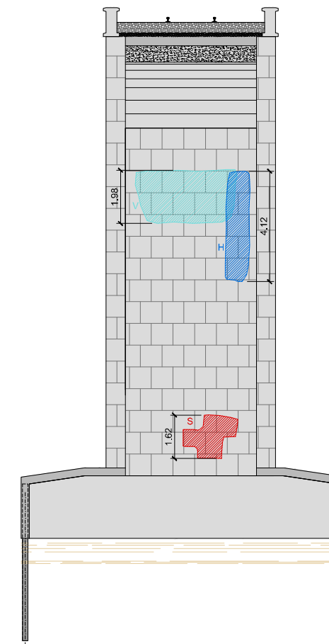
SECCIÓN P4-MUNDAKA ESCALA 1:100
