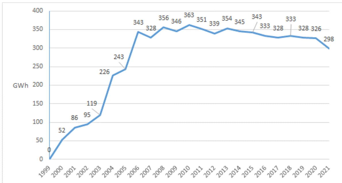
8. grafikoa. Ekoizpen elektriko eolikoaren bilakaera Euskadin (GWh; 1998-2021).
