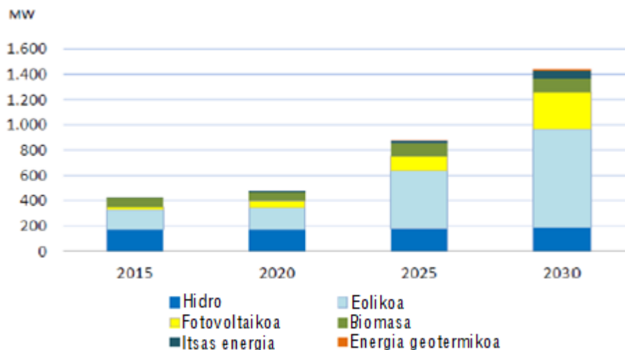
23. grafikoa. Euskadin instalatutako potentzia elektriko berriztagarriaren egoera
