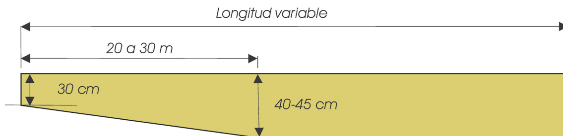
Figura 11.2. Esquema de sección longitudinal en el lecho de frenado
