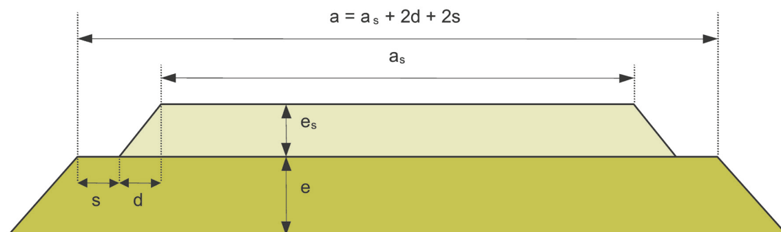
Figura 12.1. Esquema de disposición transversal del firme
