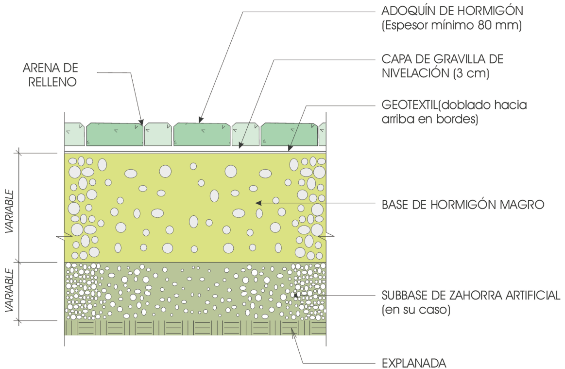
Figura 11.1. Sección de firmes con pavimento de adoquines
