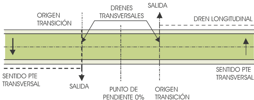
Figura 12.5. Disposición de drenes en zonas de transición de peralte
