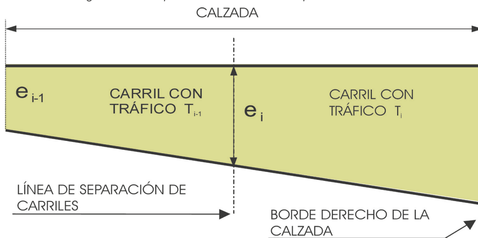
Figura 12.2. Esquema de variación de espesor entre carriles
