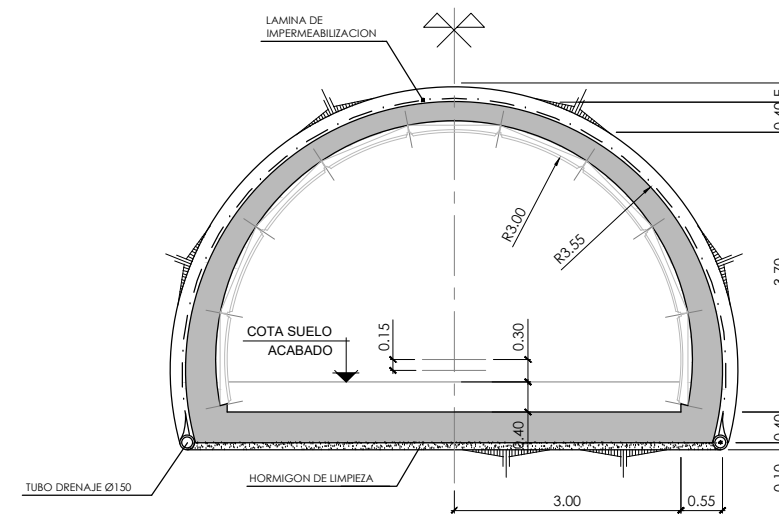
SECCION TIPO C2
