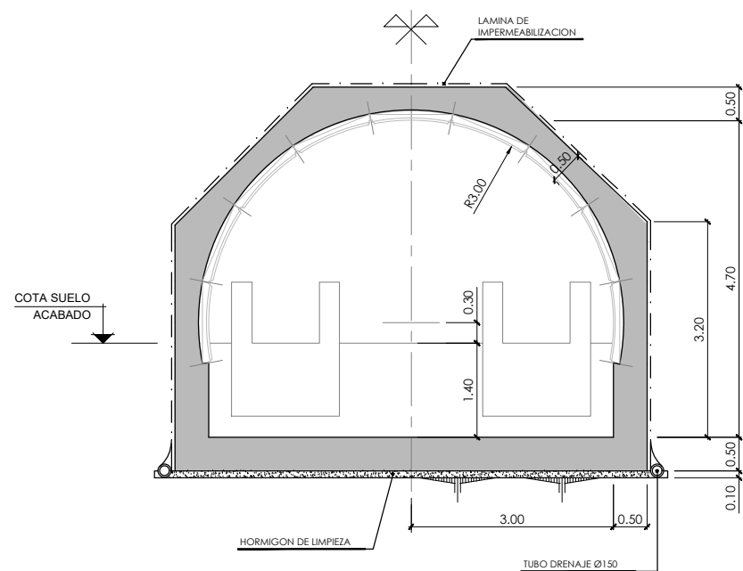
SECCION TIPO C3
