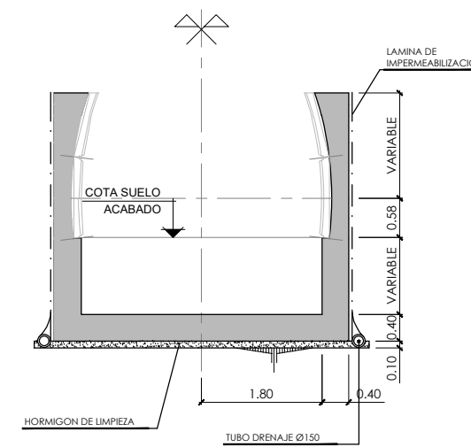
SECCION TIPO C6
