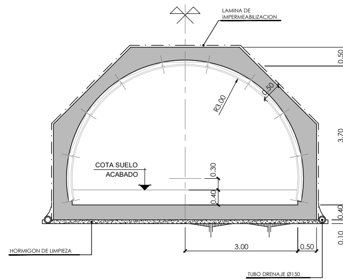
SECCION TIPO C4
