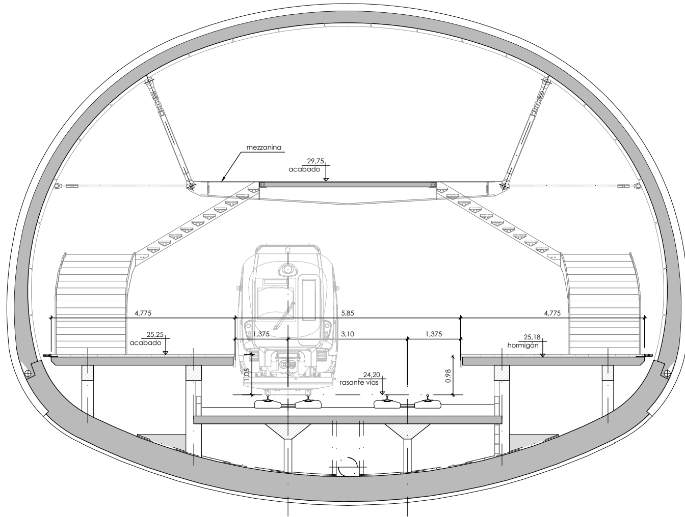
SECCIÓN TIPO POR ANDÉN
