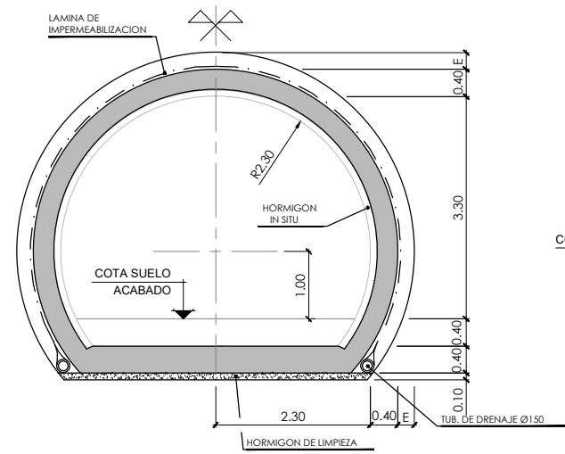
SECCION TIPO C0
