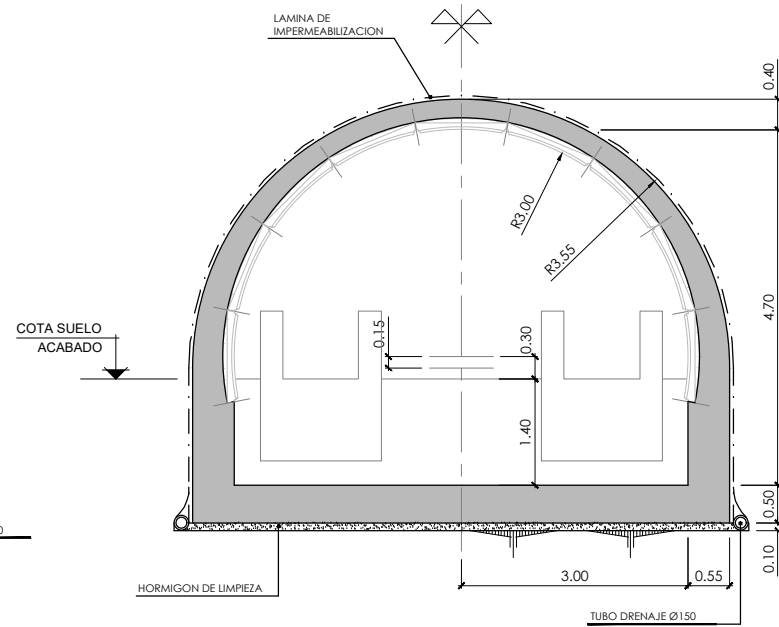
SECCION TIPO C1
