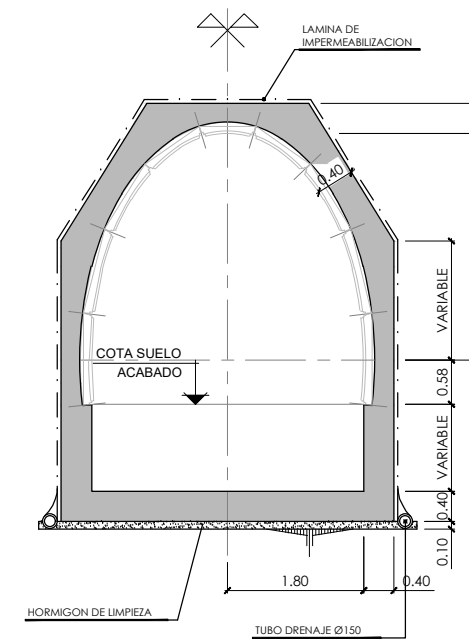
SECCION TIPO C5
