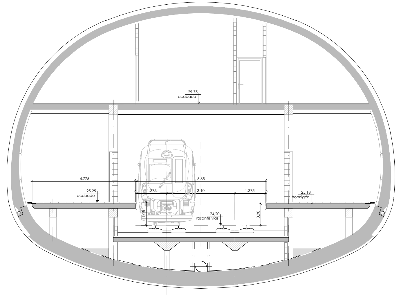
SECCIÓN TIPO POR CUARTOS TÉCNICOS
