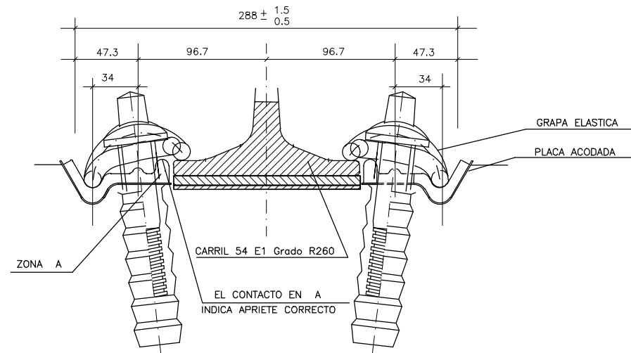
ELEMENTOS DE LA SUJECCION ESCALA 1:2
