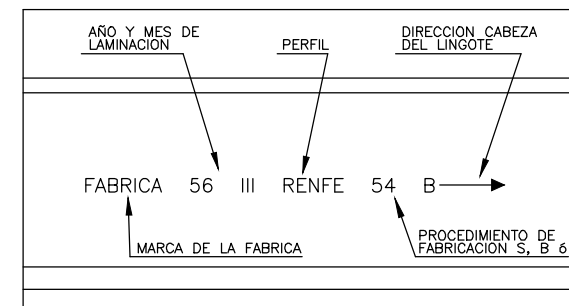
MARCAS DE FABRICACION ESCALA 1:2
