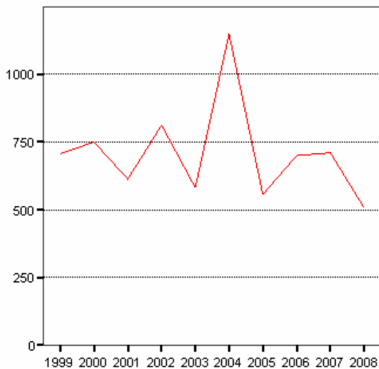
Figura 1.8- Tasas de incidencia de varicela por 100.000 habitantes. Álava 1999-2008.
