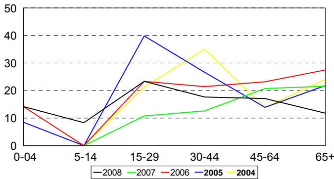
Figura 1.11- Tasas TBC/100.000 habitantes por grupos de edad. Álava 2004-2008.
