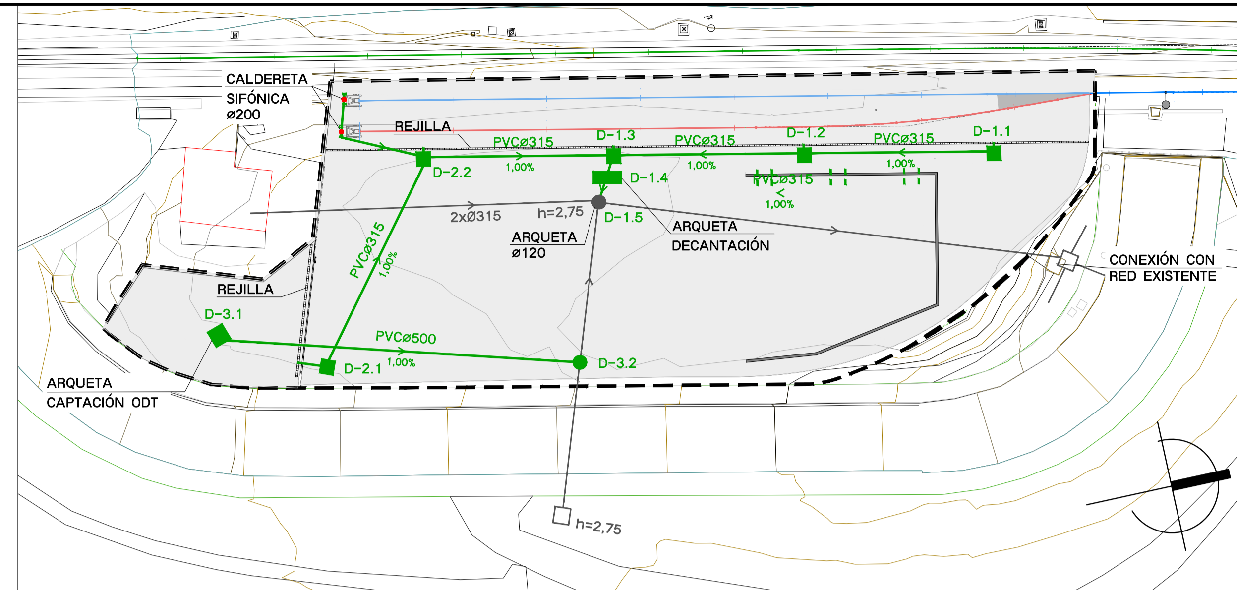
PLANTA E 1/400
