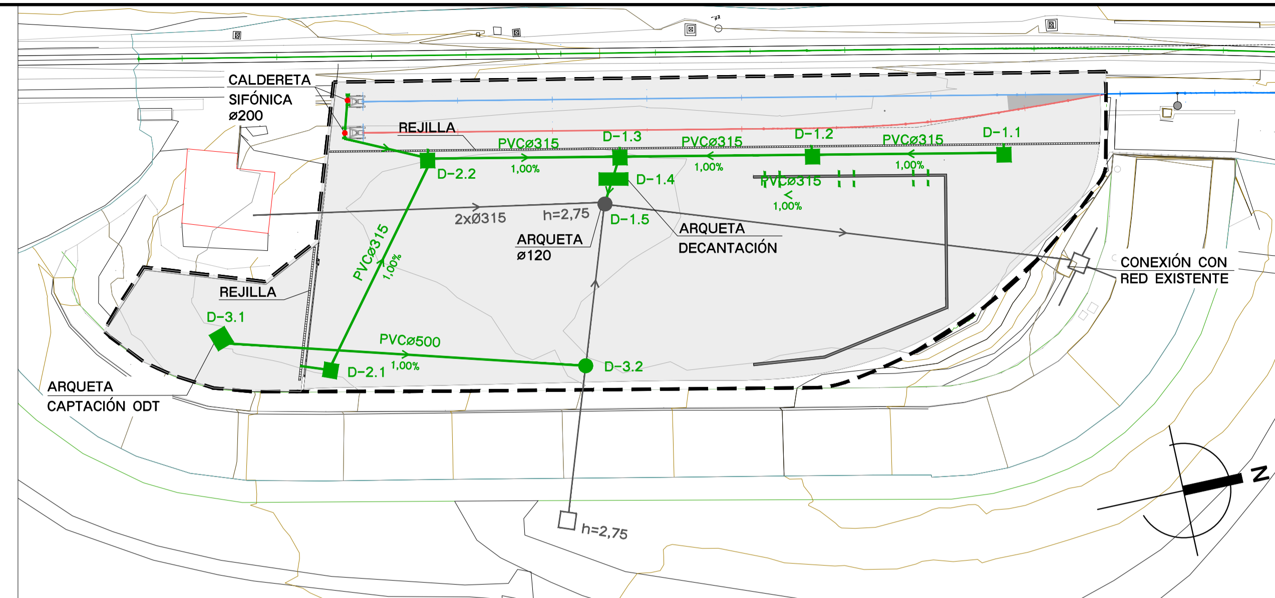
PLANTA E 1/400
