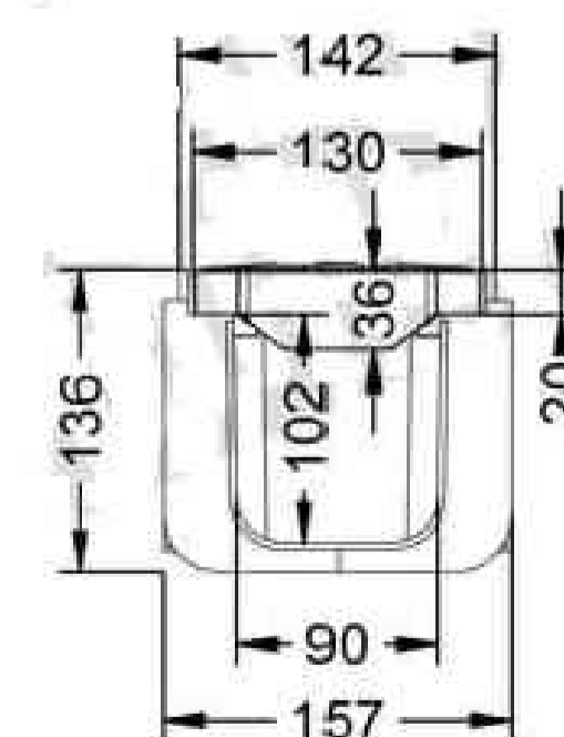
CONJUNTO CANAL POLIPROPILENO Y REJILLA COMPOSITO 157X781mm D400
