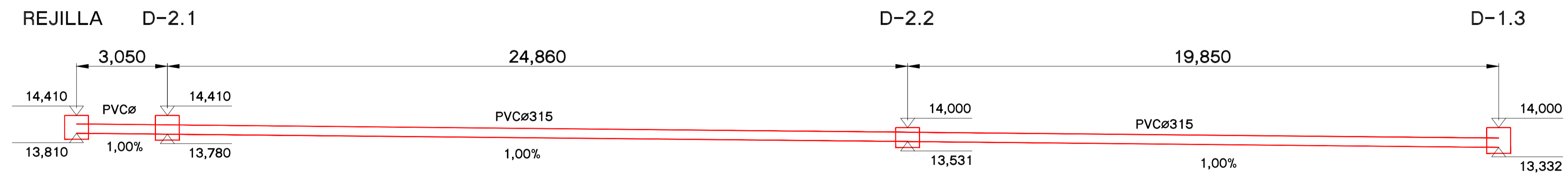
EJE 2 E 1/100
