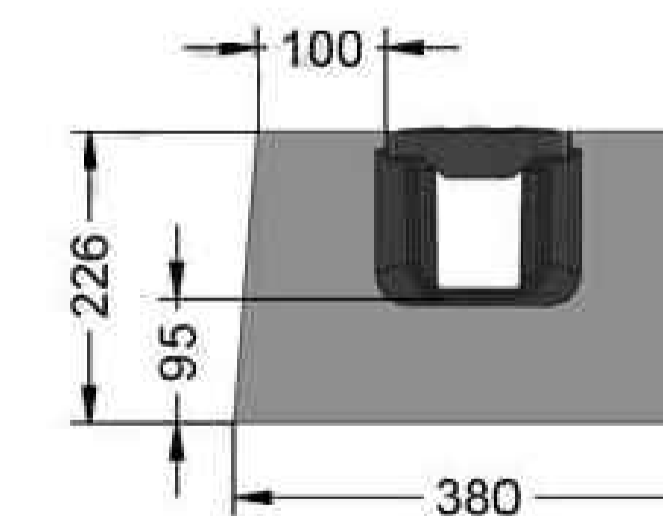
BASE DE HORMIGÓN (H30) PARA CIMENTACIÓN
