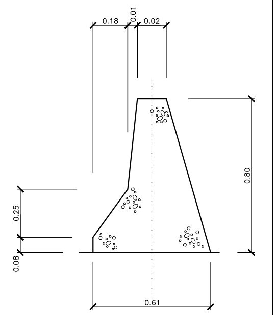
BARRERA DE HORMIGON SIMPLE PERFIL NEW JERSEY. BHSPJ3/1a. ESCALA 1/10
