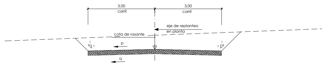
SECCIÓN TIPO DEL Pk. 0+000,000 AL 0+035,000 ESCALA 1:50
