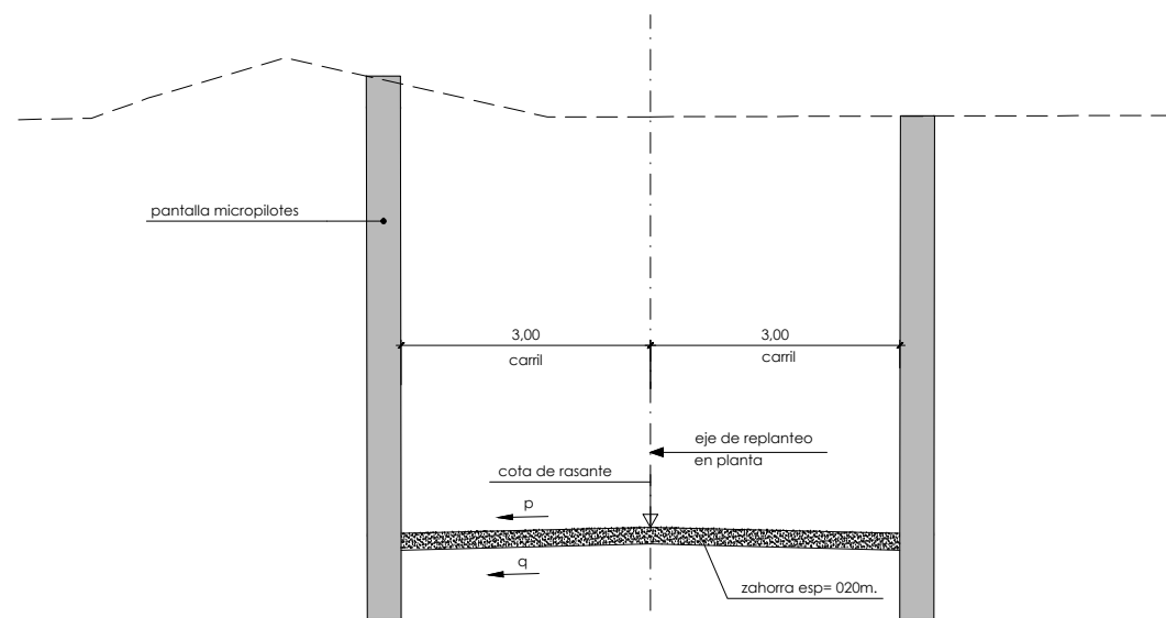
SECCIÓN TIPO DEL Pk. 0+057,000 AL 0+104,000 ESCALA 1:50
