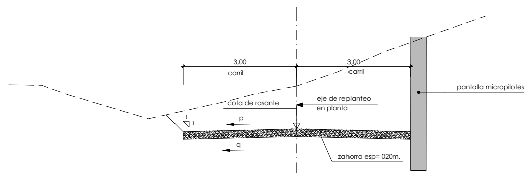
SECCIÓN TIPO DEL Pk. 0+035,000 AL 0+057,000 ESCALA 1:50
