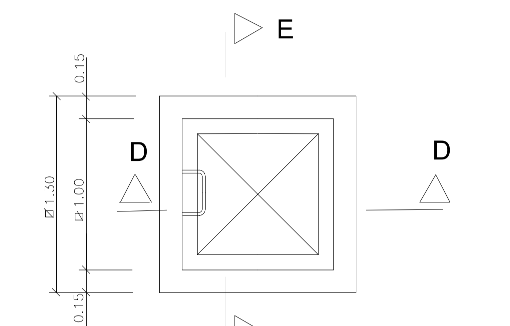
PLANTA ARQUETA PARA VENTOSA ESCALA 1:25
