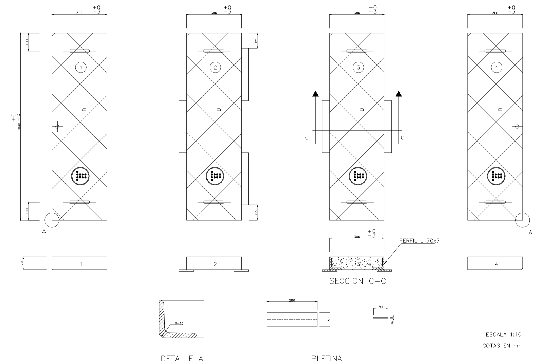
TAPA PARA ARQUETA TIPO D CONSTRUIDA "IN SITU"
