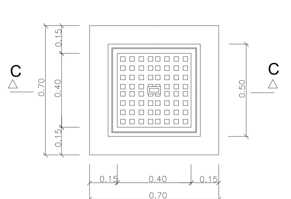
PLANTA ARQUETA PARA ACOMETIDAS ESCALA 1:10
