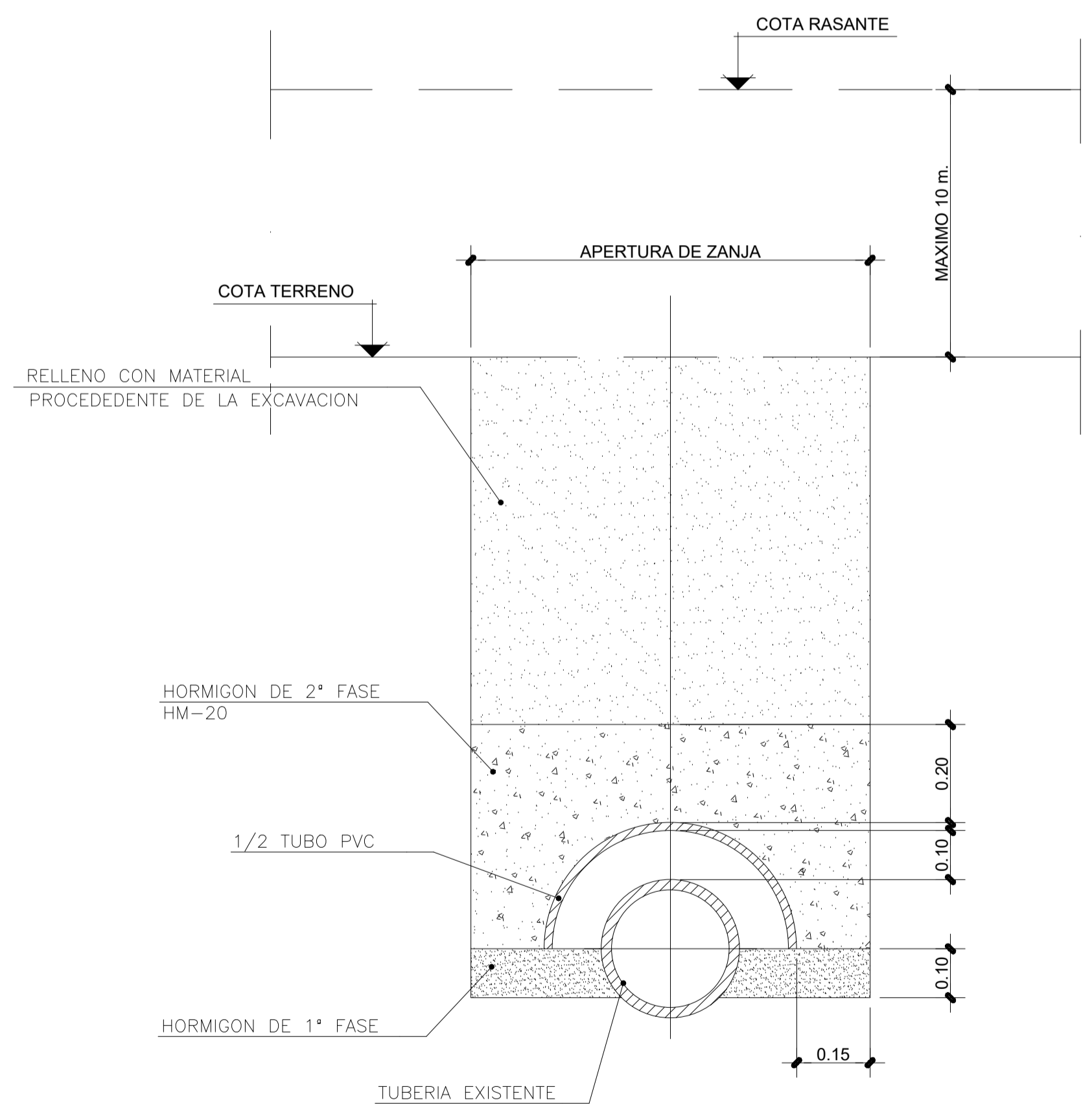
DETALLE DE REFUERZO DE TUBERIA BAJO CALZADA ESCALA 1/10
