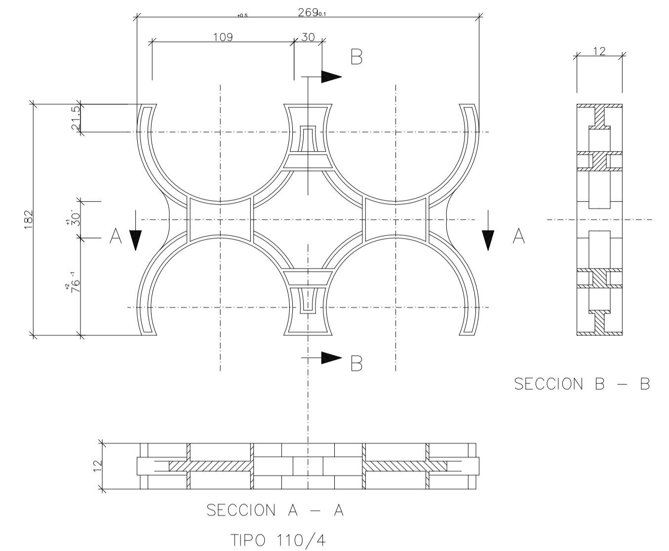
SOPORTES DISTANCIADORES
