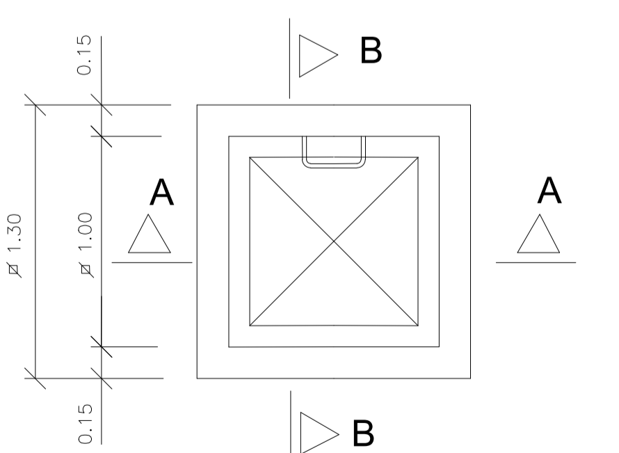
PLANTA ARQUETA PARA VALVULAS ESCALA 1:25
