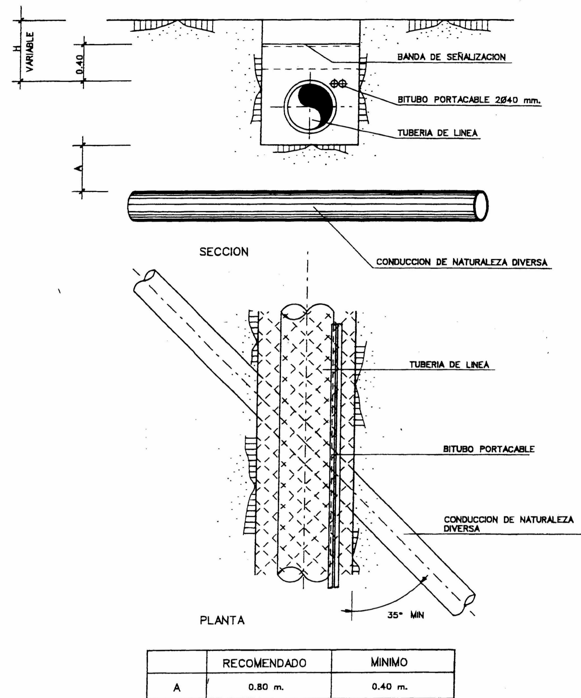
CRUCE CON CONDUCCIONES DE NATURALEZA DIVERSA ESCALA 1/40
