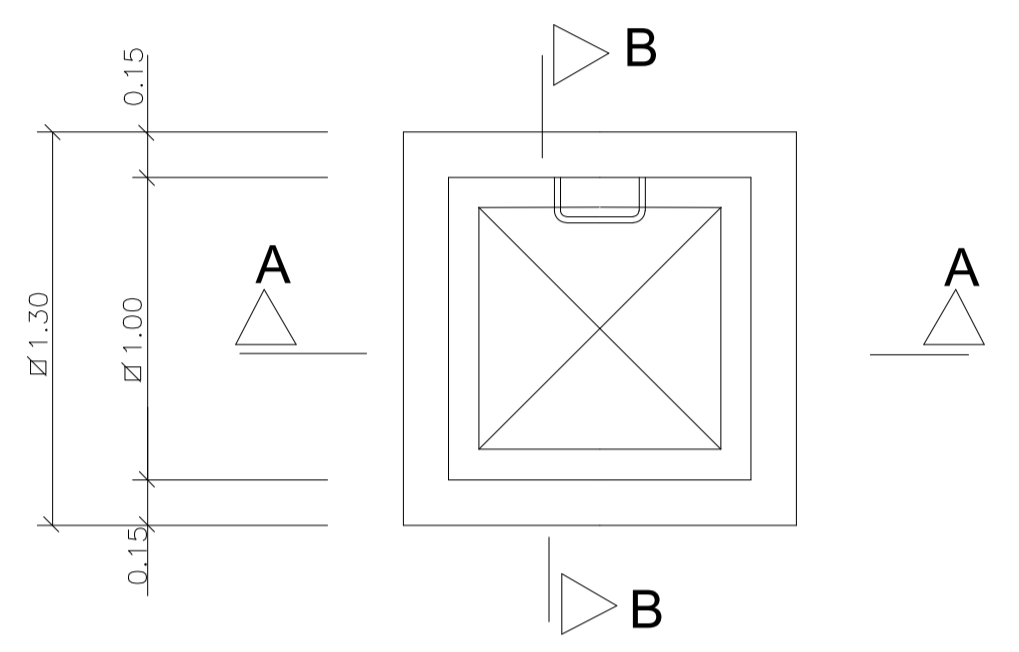
PLANTA ARQUETA TIPO ESCALA 1:25
