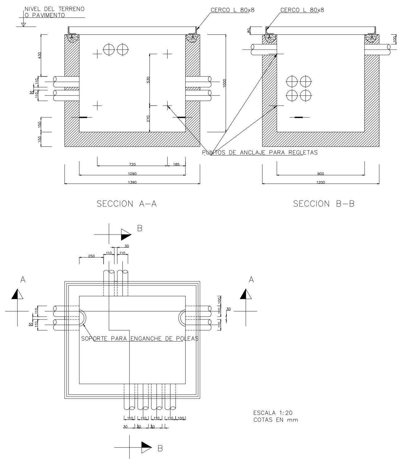
ENTRADA DE CONDUCTOS Ø63 POR PARED TRANSVERSAL
