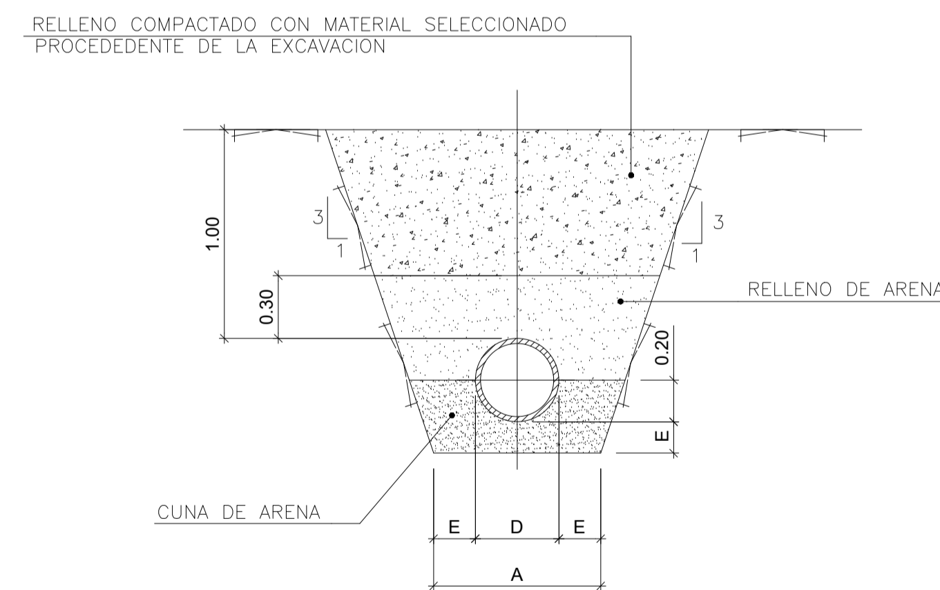
ALojAMIENTO PARA TUBERIA SIN PREZANJA
