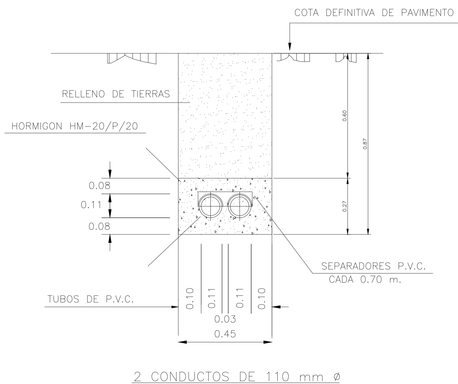
ZANJAS TIPO Y CANALIZACIONES
