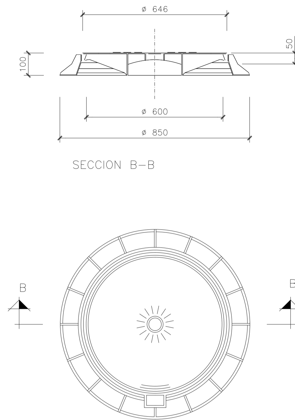
PLANTA
