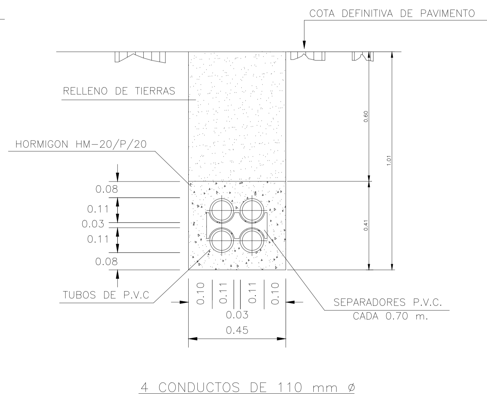
ZANJAS TIPO Y CANALIZACIONES
