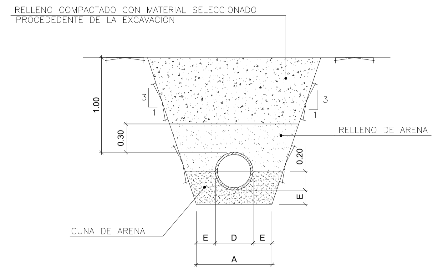
ALOJAMIENTO PARA TUBERIA SIN PREZANJA ESCALA 1/25
