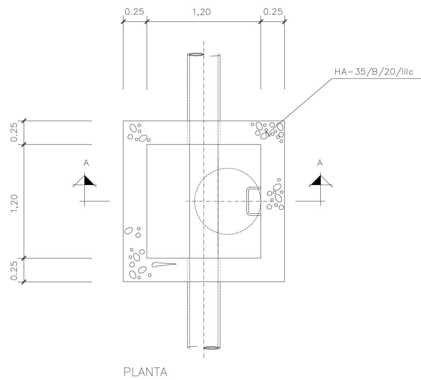
PLANTA
