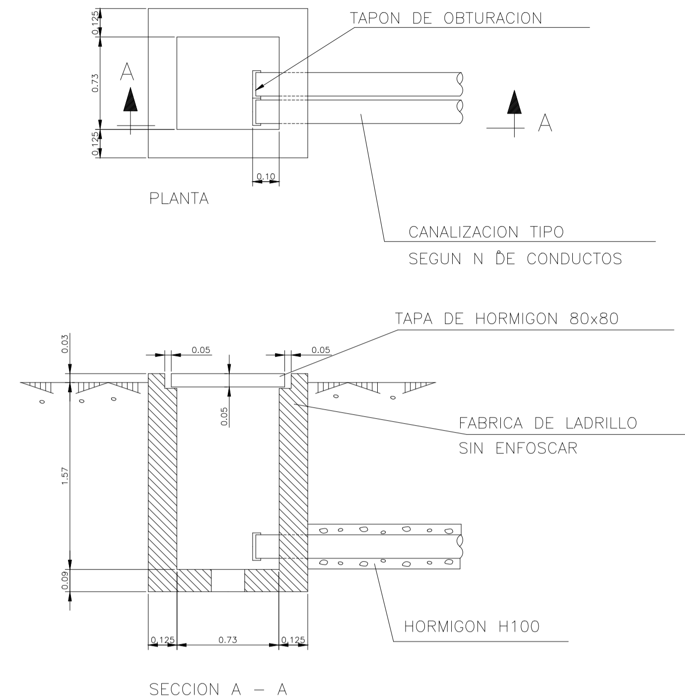
ARQUETA PROVISIONAL FINAL CANALIZACION
