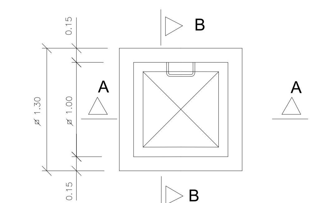
PLANTA ARQUETA PARA DESAGUE ESCALA 1:25
