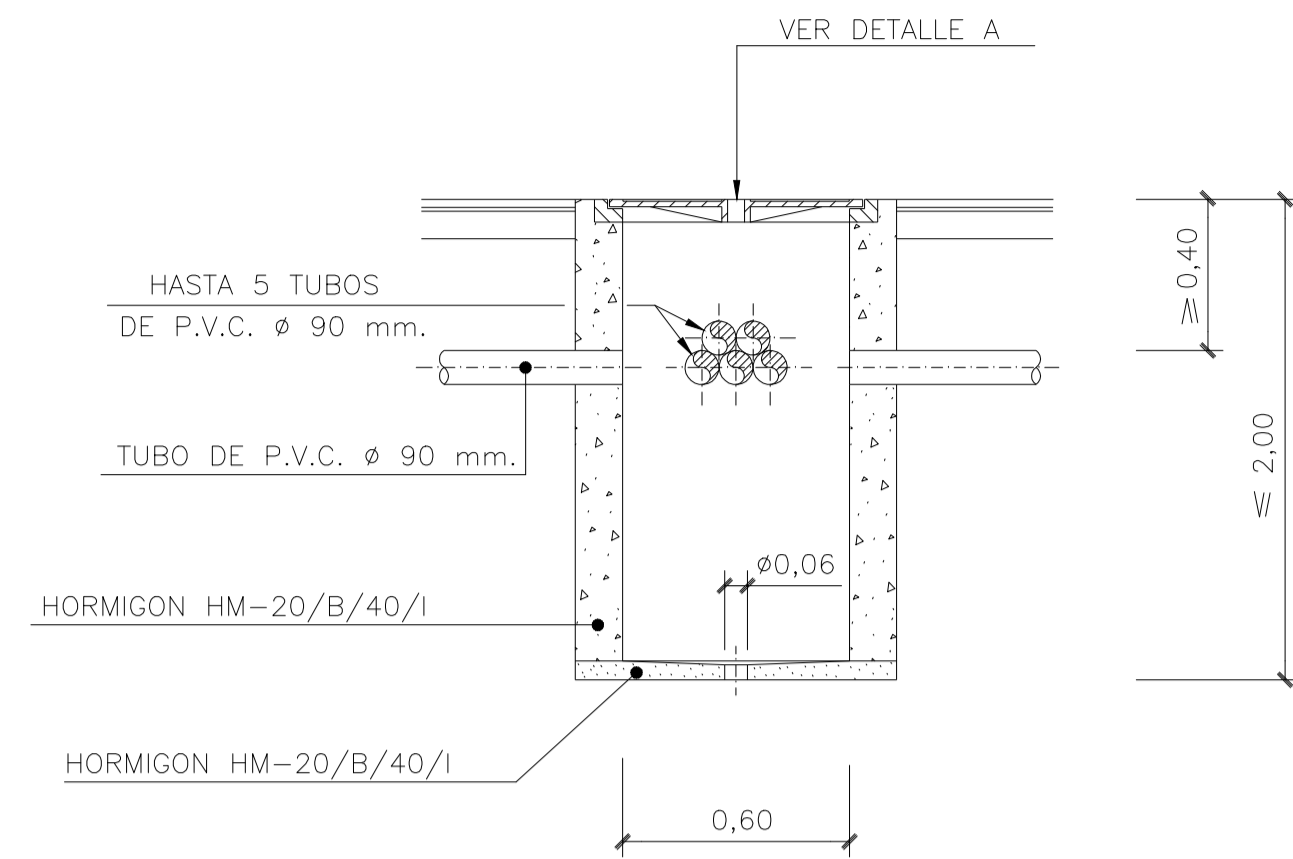
ARQUETA PARA DERIVACIONES, ACOMETIDAS O CRUCE DE CALZADA ESCALA 1/20
