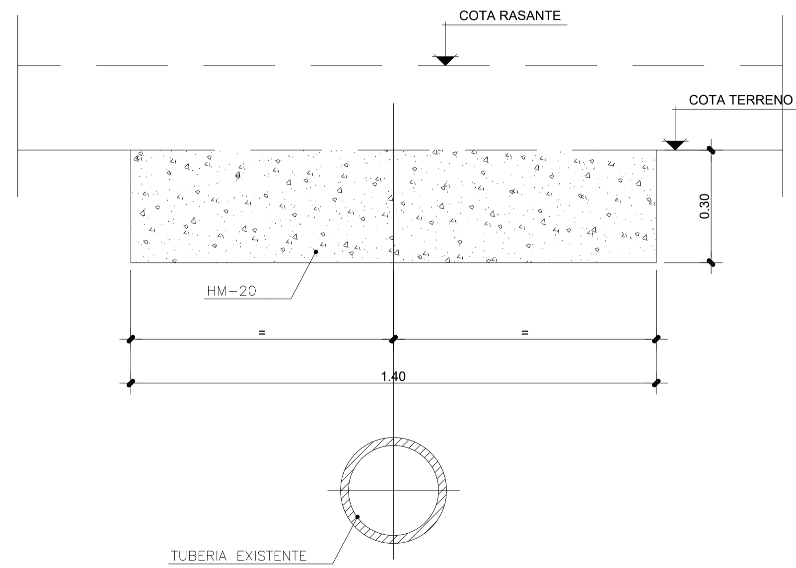
DETALLE DE REFUERZO DE TUBERIA BAJO CALZADA < 2 m. ESCALA 1/10
