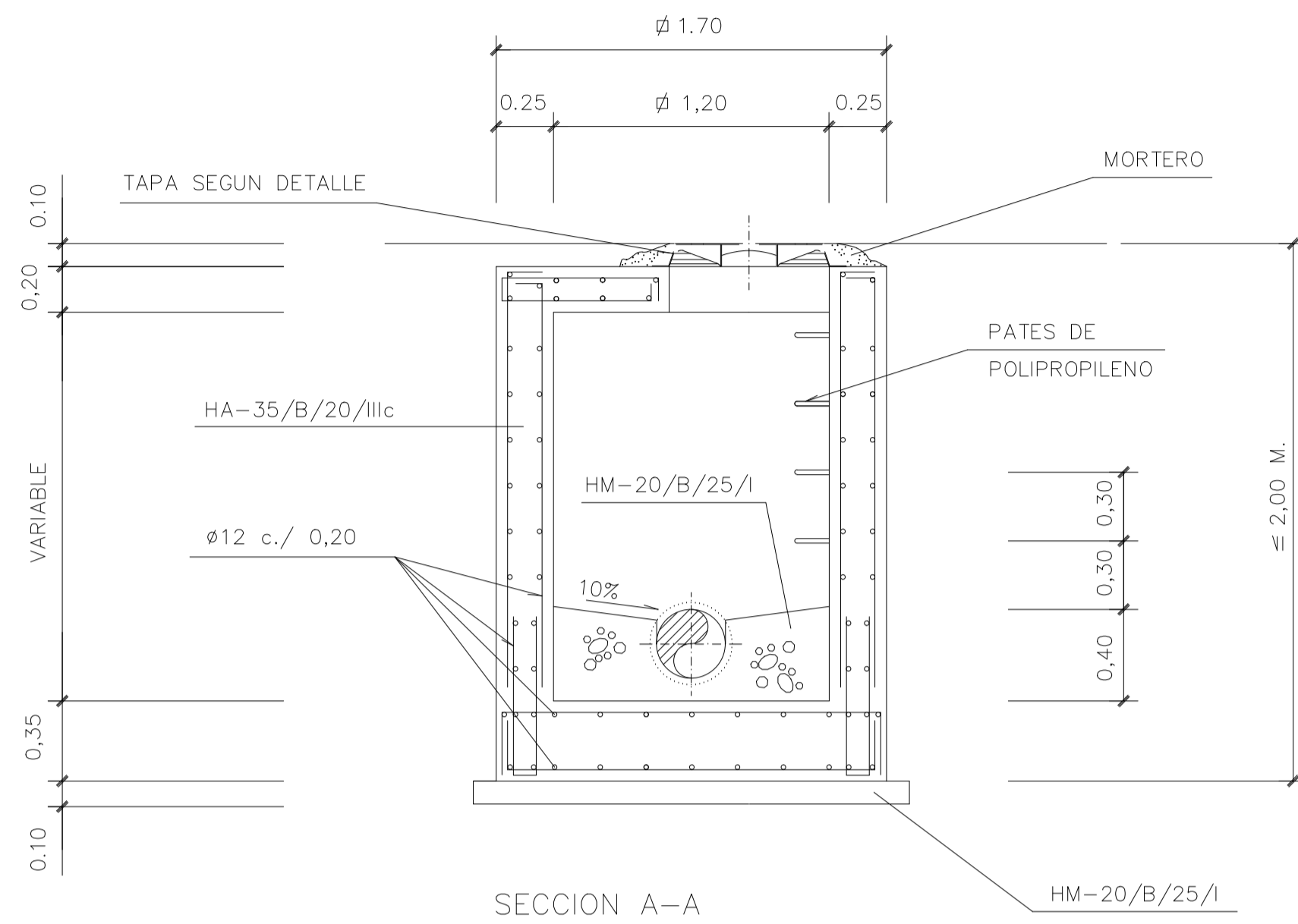
SECCION A-A
