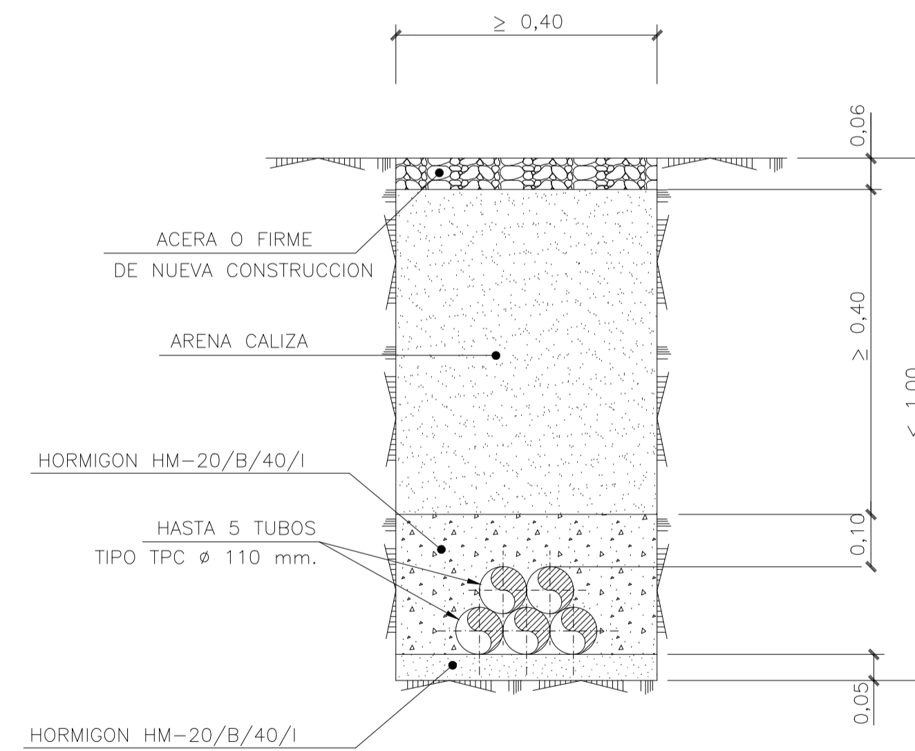
CANALIZACION ELECTRICA EN ZANJA BAJO ACERA DE NUEVA CONSTRUCCION, EN CRUCES Y FUERA DE ZONA DE OBRAS ESCALA 1/10
