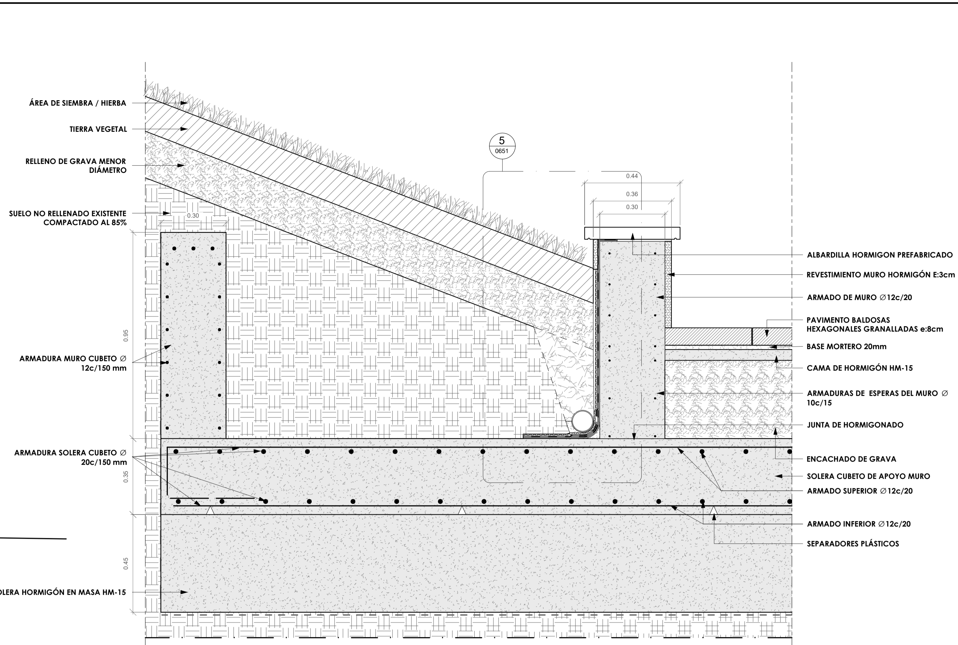
4 DETALLE MURO APOYADO EN SOLERA ESCALA: 1 : 10
