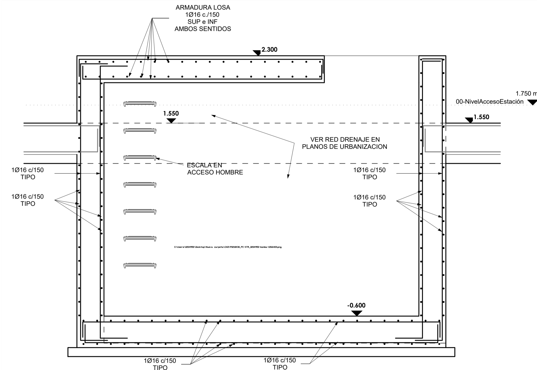
2 SECCION ESCALA: 1 : 20
