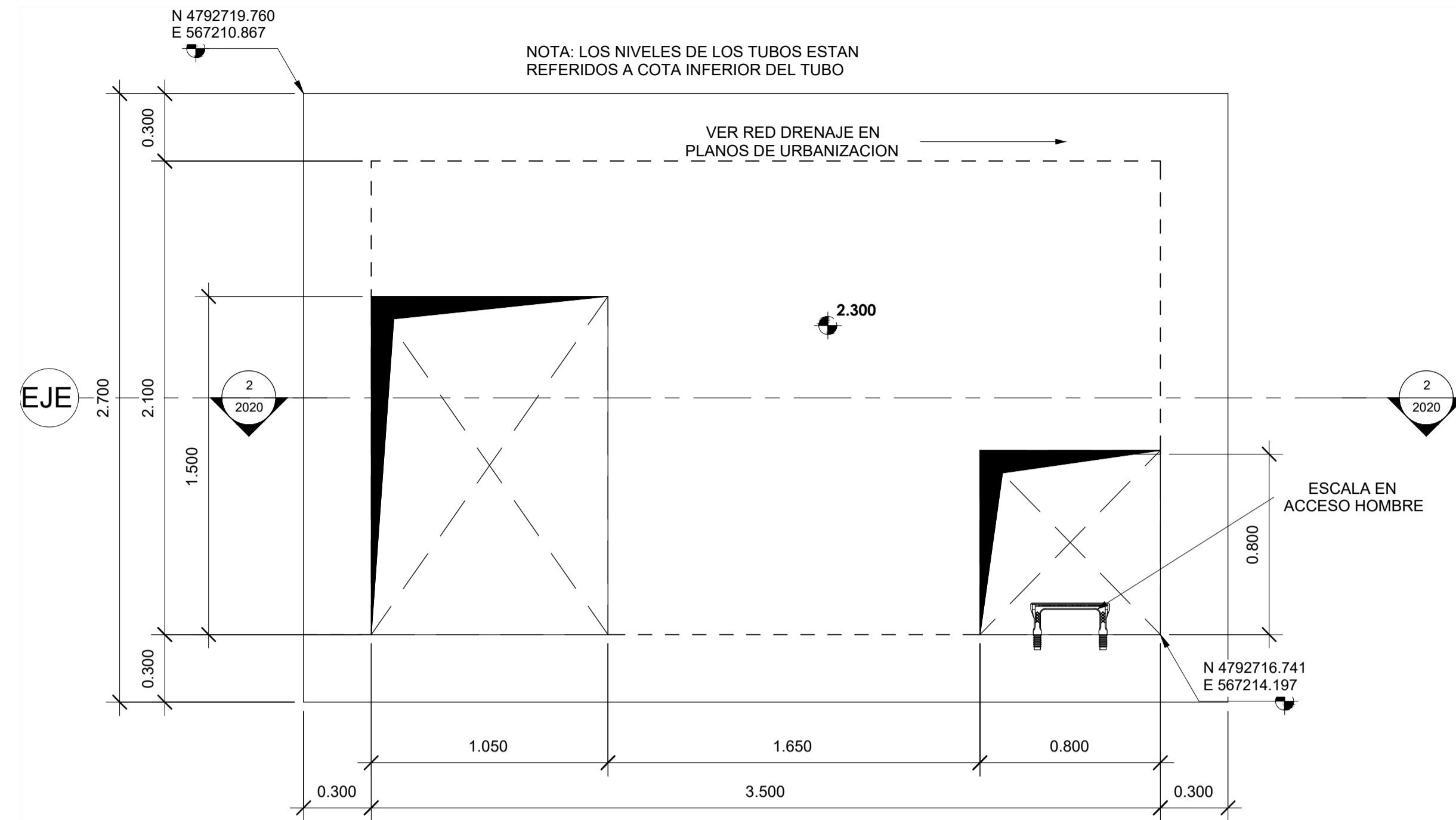
1 PLANTA ESCALA: 1 : 20
