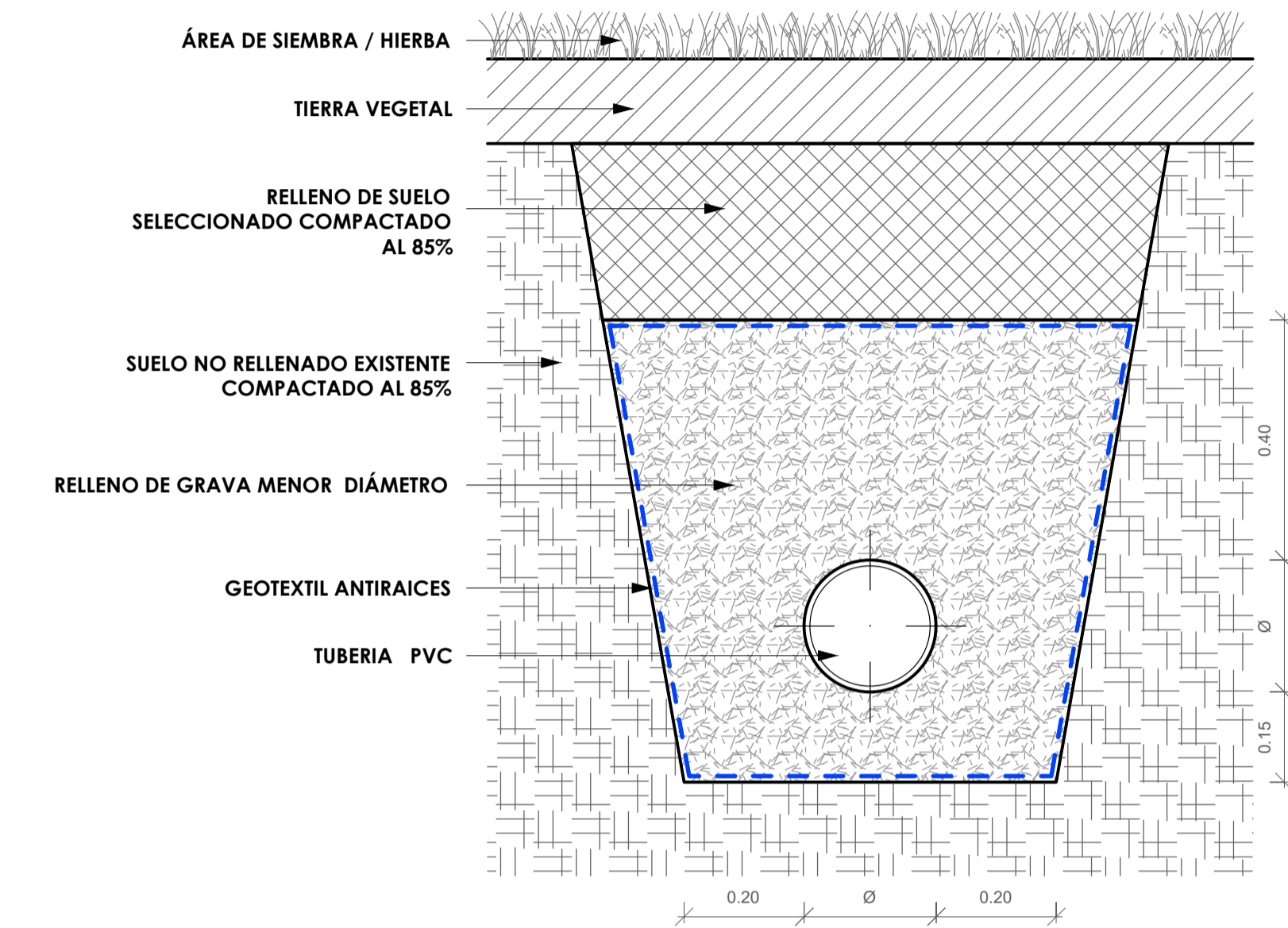
2 ZANJAS DRENAJE SOBRE COTA +2.50 ESCALA: 1 : 10
