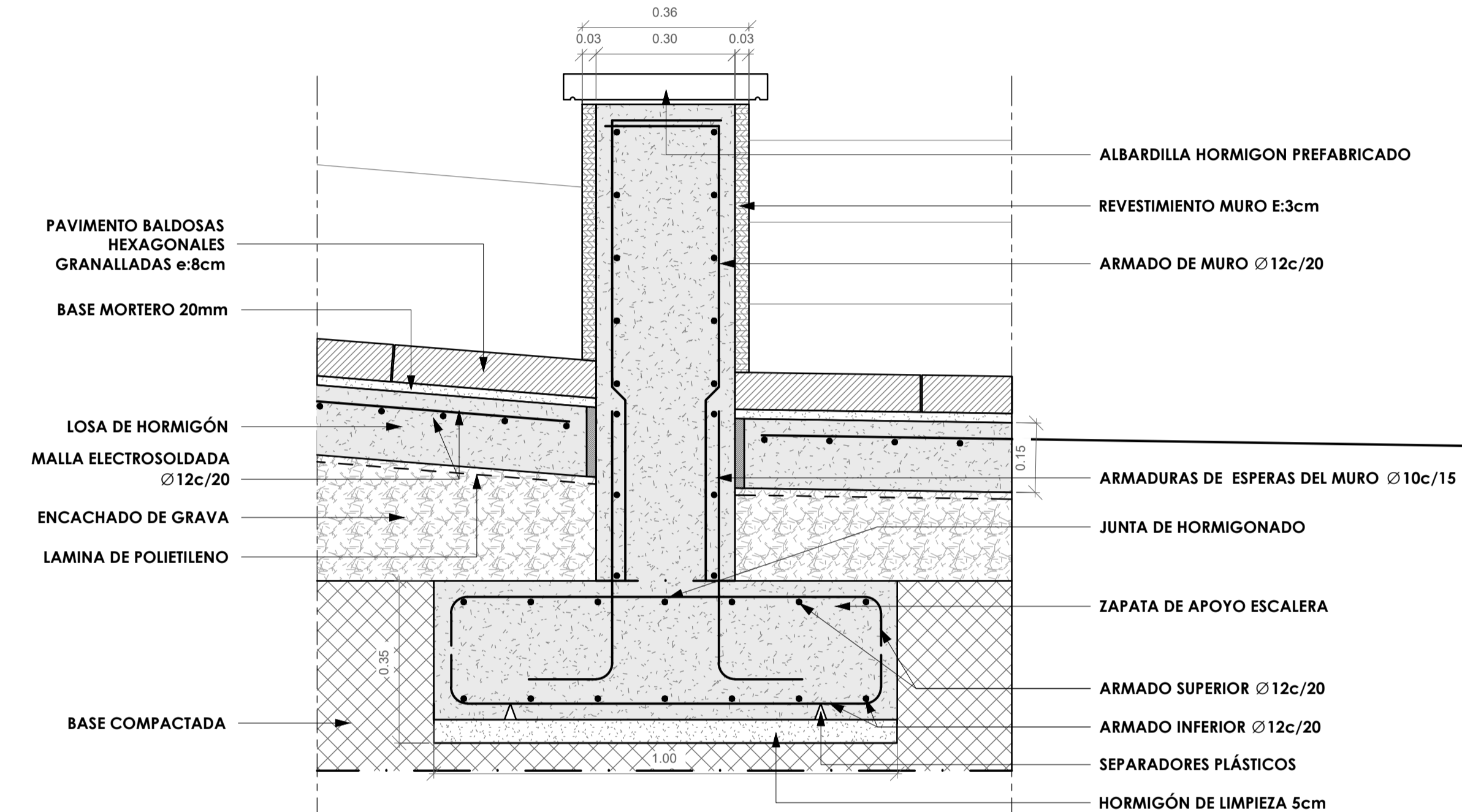
2 DETALLE MURO APOYADO EN ZAPATA ESCALA: 1 : 10
