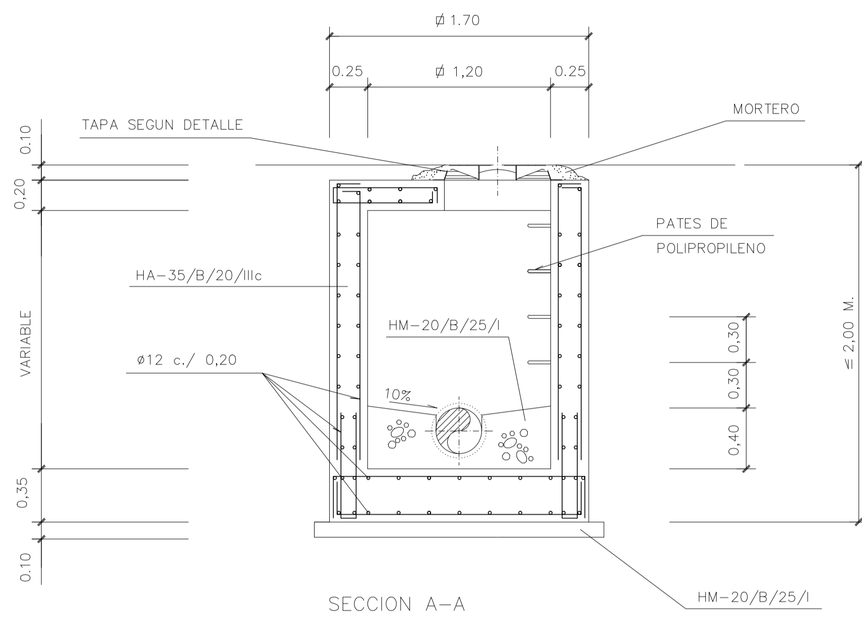
SECCION A-A
