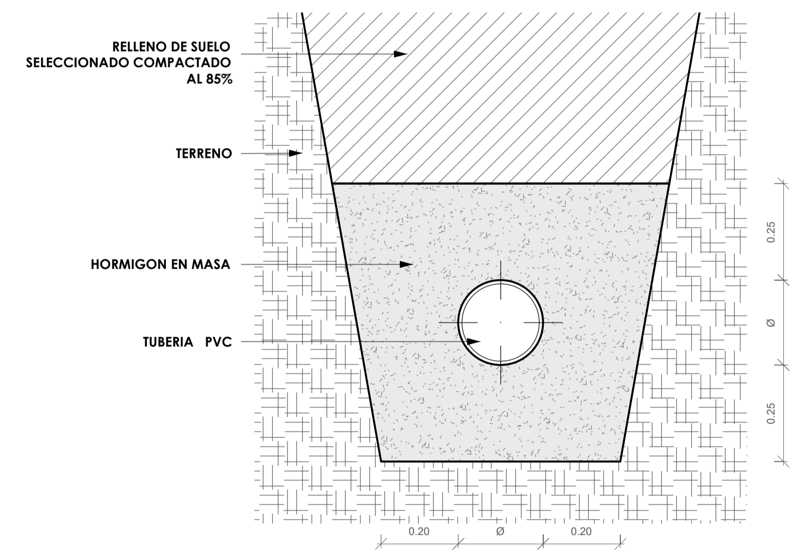
3 ZANJAS DRENAJE BAJO COTA +2.50 ESCALA: 1 : 10
