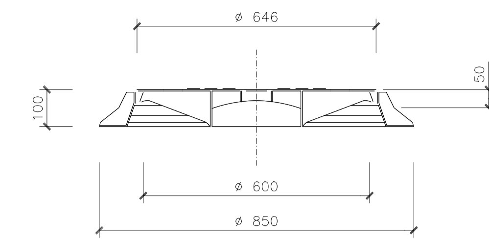
SECCION B-B
