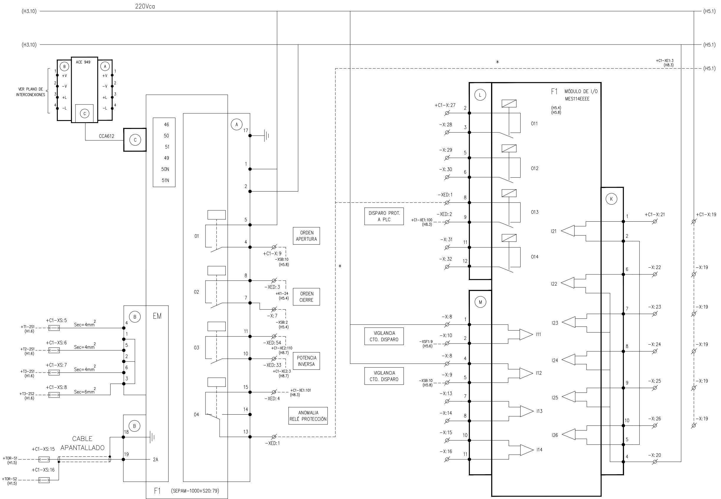
RELÉ PROTECCIÓN TIPO SEPAM-1000 E INTERFACE COMUNICACIÓN CON PLC ACE949 MÓDULO DE ENTRADAS / SALIDAS ADICIONALES PARA SEPAM 1000 EN Vcc
