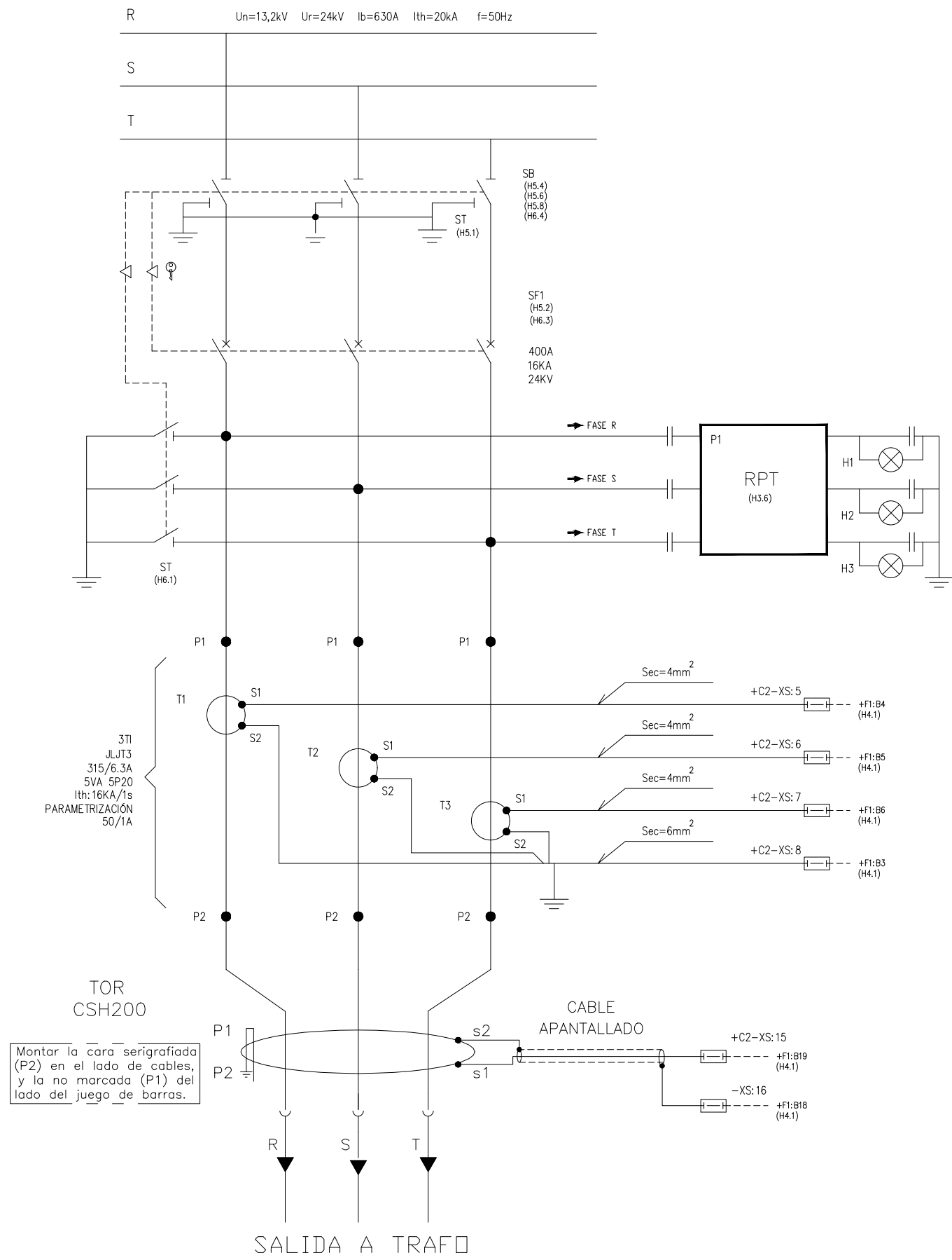
+A1.C2 CIRCUITO DE POTENCIA
