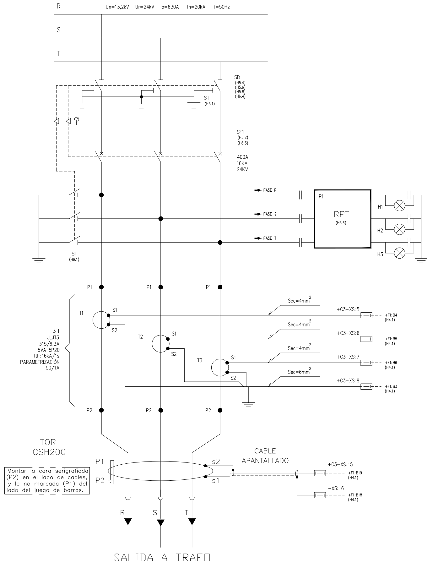
+A1.C3 CIRCUITO DE POTENCIA
