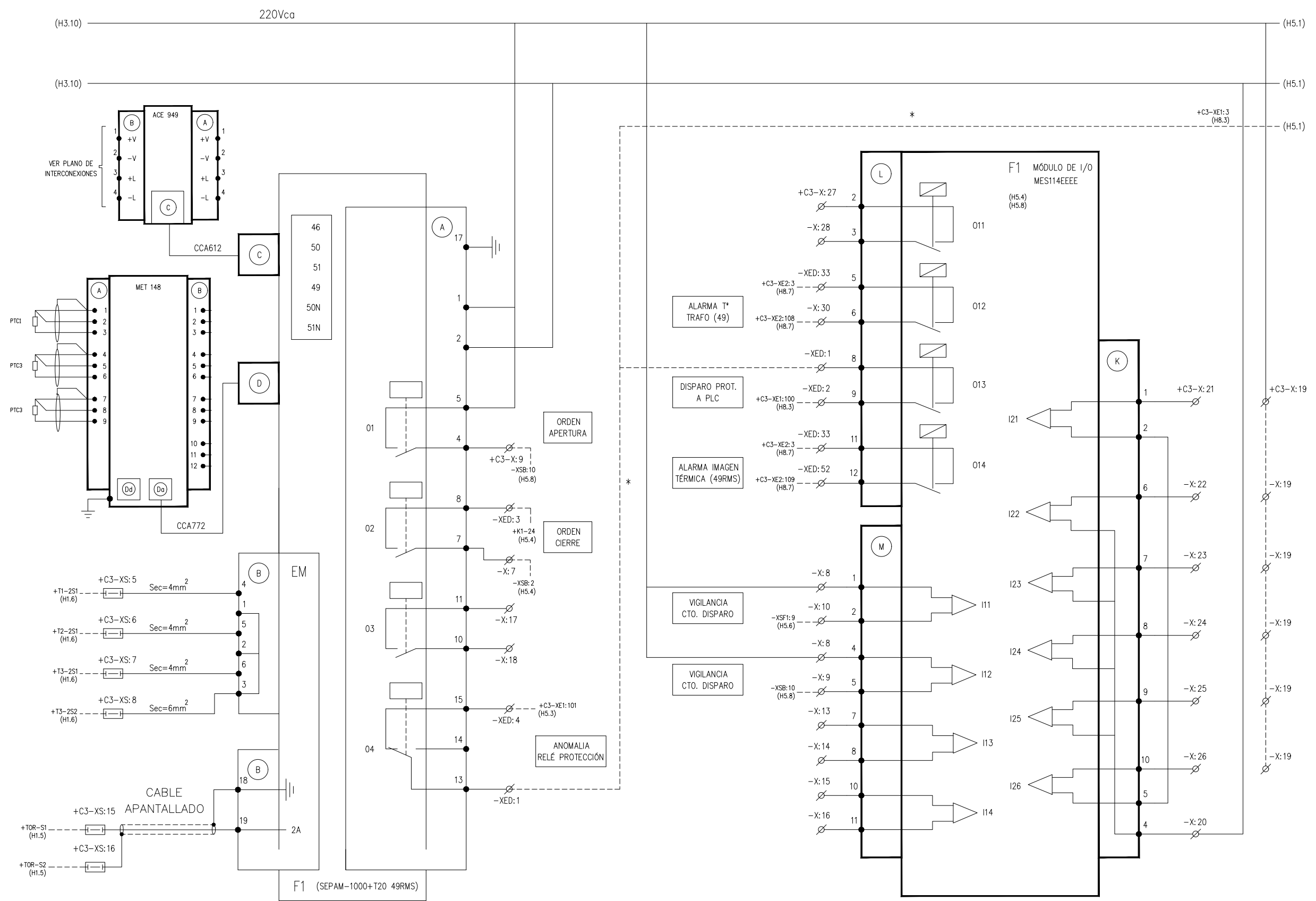
RELÉ PROTECCIÓN TIPO SEPAM-1000 E INTERFACE COMUNICACIÓN CON PLC ACE949
