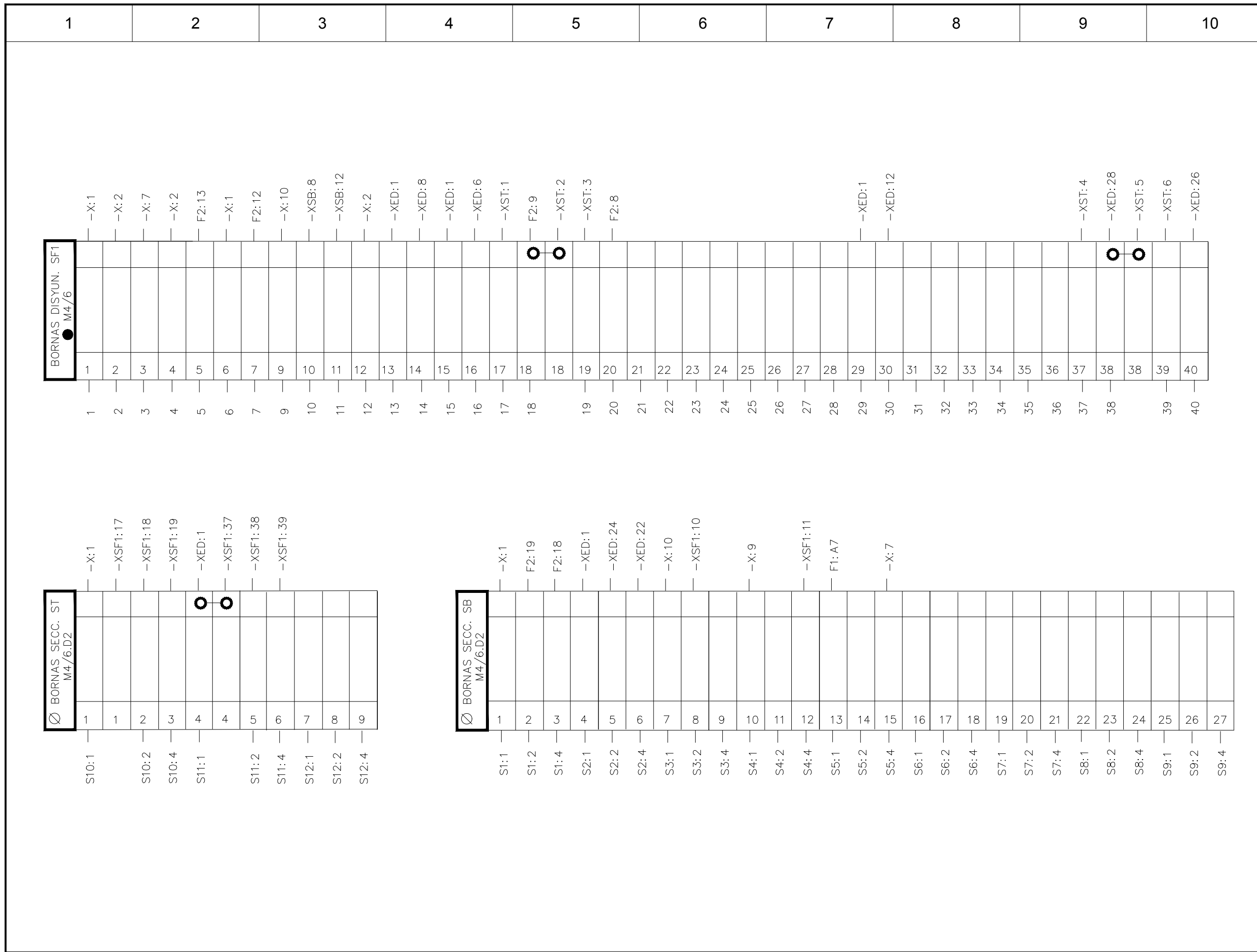
+A1.C1 BORNEROS DISYUNTOR (SF1) Y SECCIONADOR DE BARRAS (SB) Y A TIERRA (ST)
