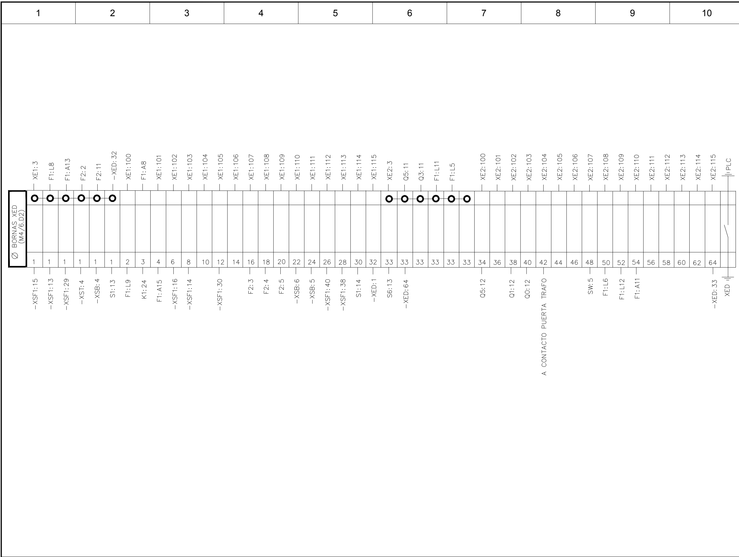
+A1.C1 BORNERO PARA TARJETAS DE ENTRADA A PLC (XED)
