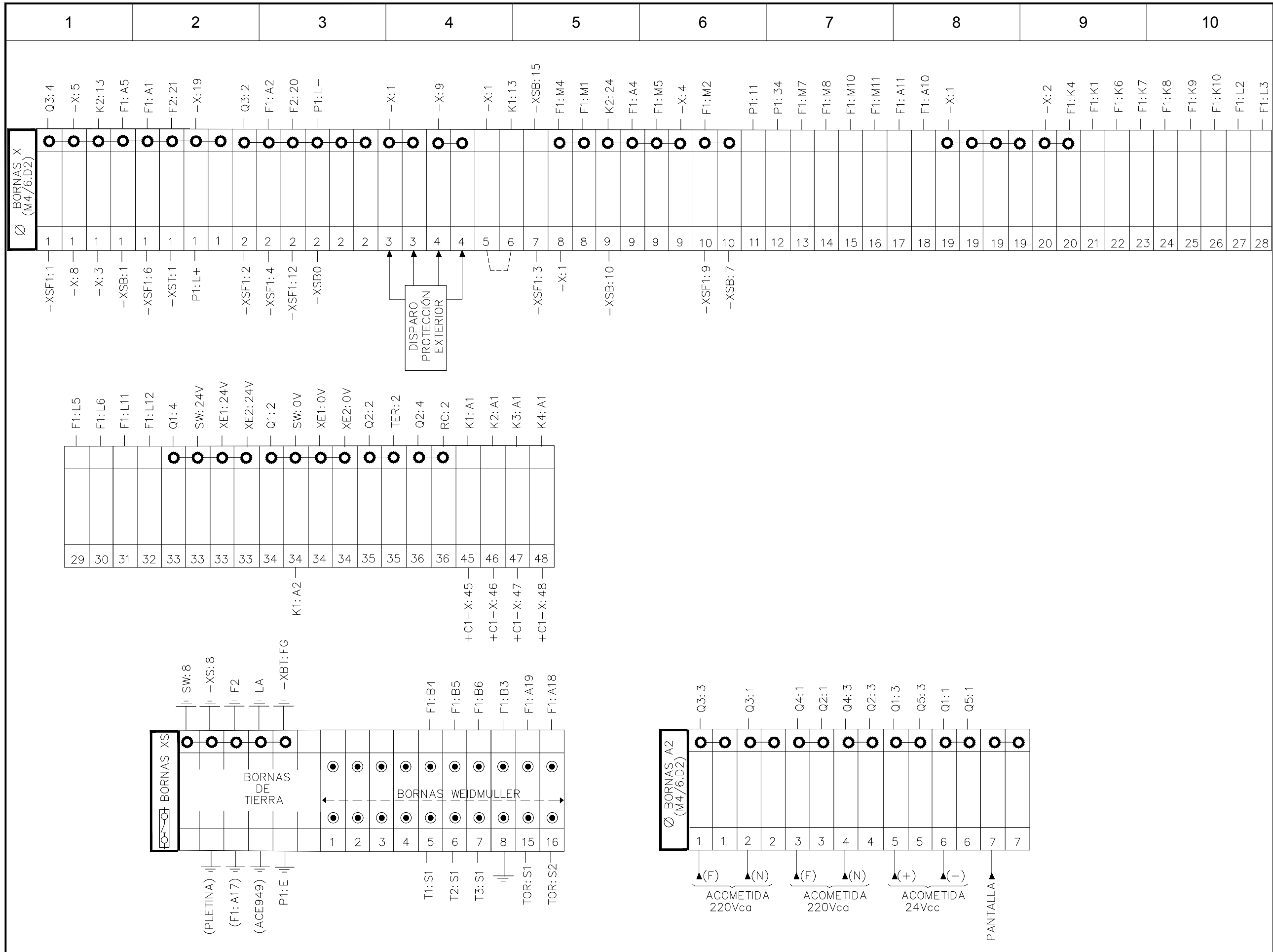
+A1.C2 BORNEROS GENERAL, SECCIONABLES (XS) Y DE ACOMETIDA DE FUERZA (A2)
