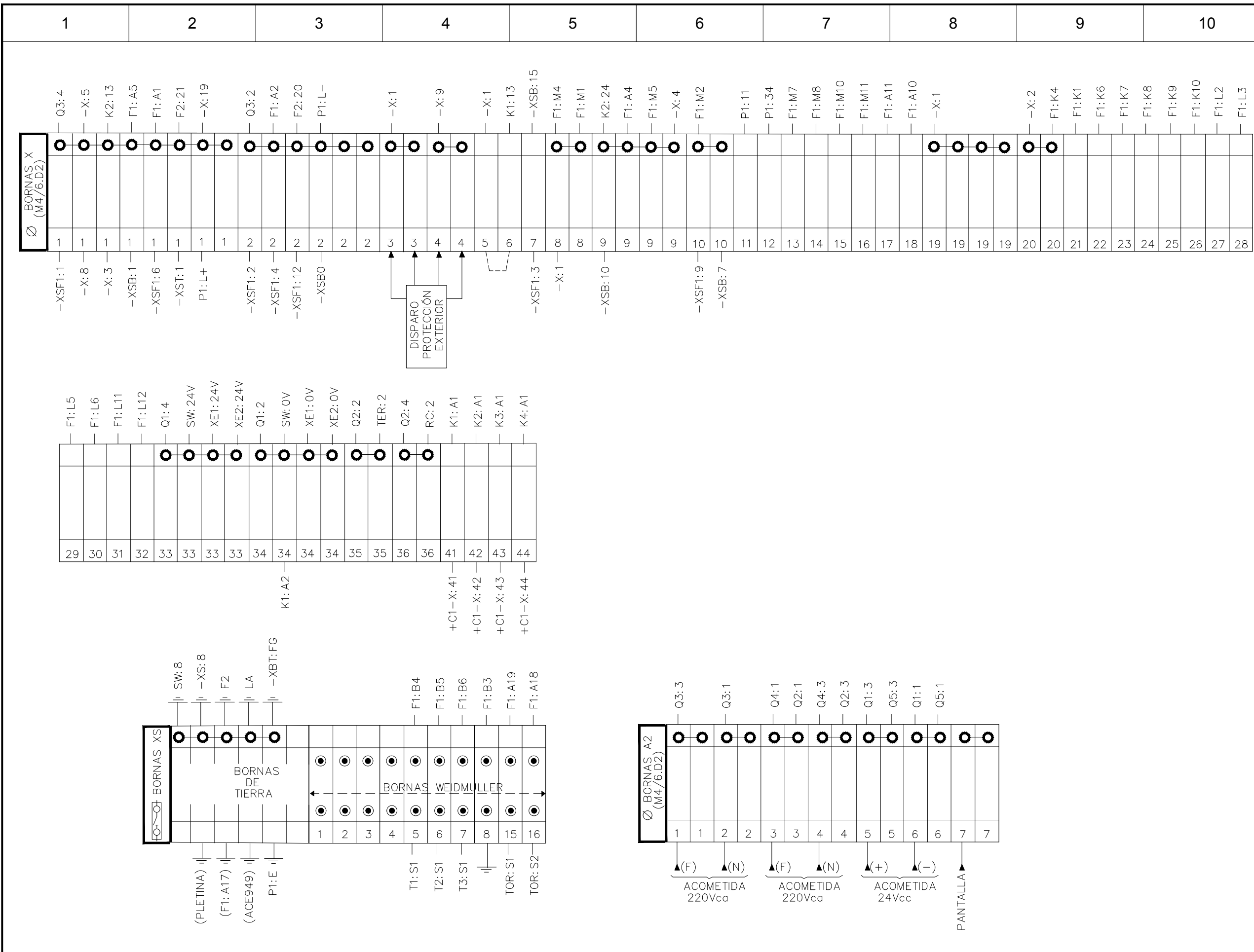
+A1.C3 BORNEROS GENERAL, SECCIONABLES (XS) Y DE ACOMETIDA DE FUERZA (A2)
