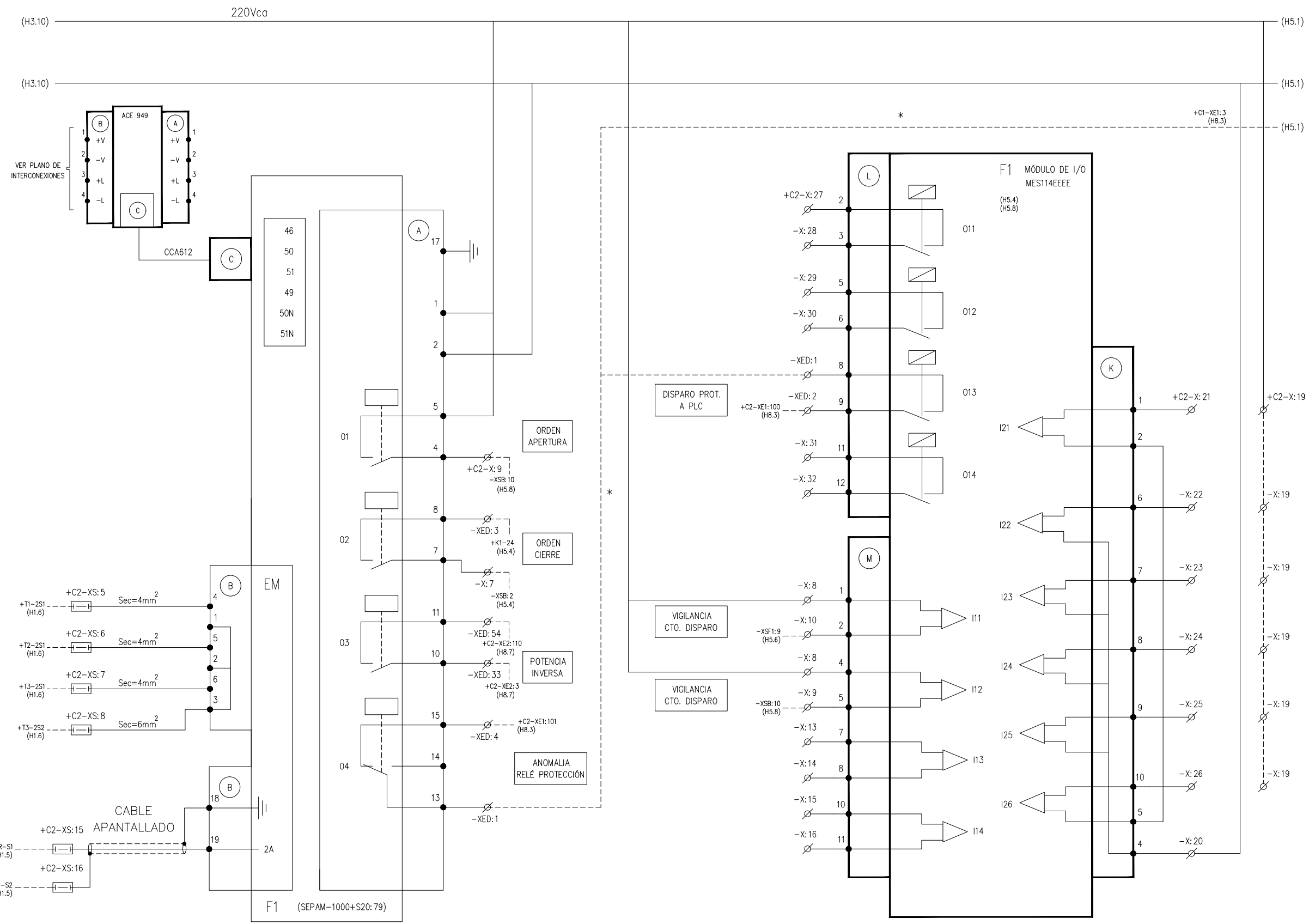
RELÉ PROTECCIÓN TIPO SEPAM-1000 E INTERFACE COMUNICACIÓN CON PLC ACE949
