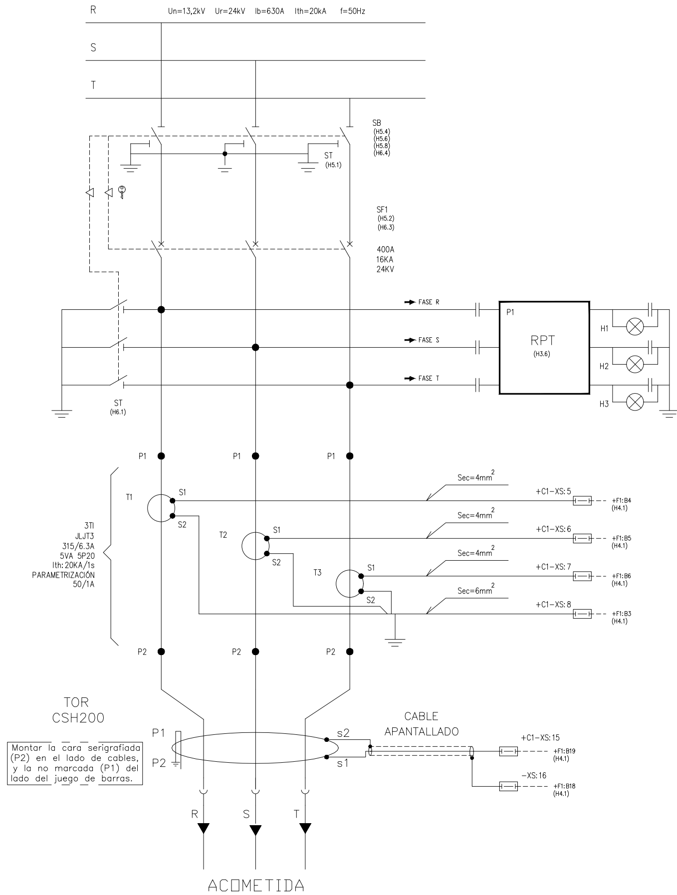
+A1.C1 CIRCUITO DE POTENCIA
