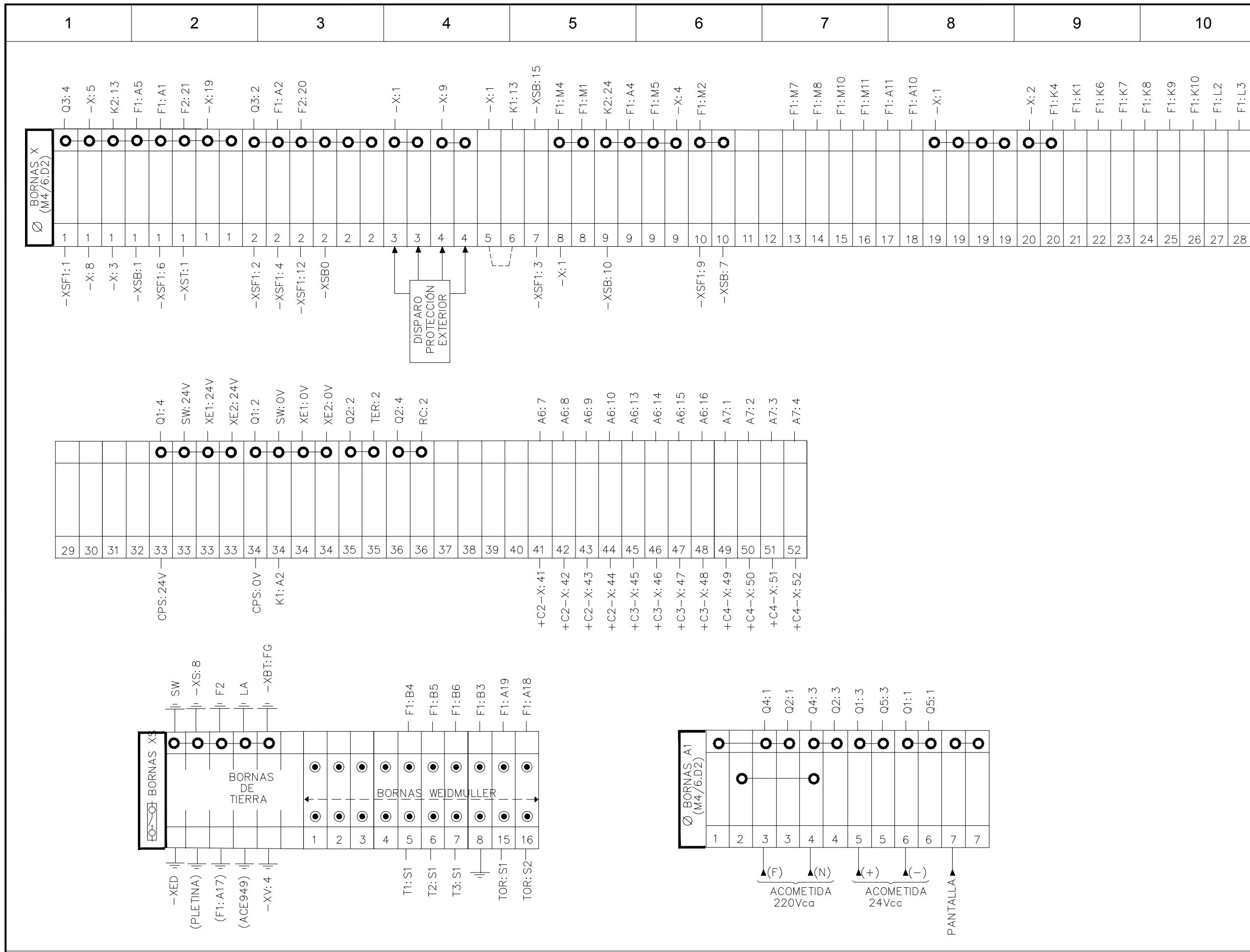
+A1.C1 BORNEROS GENERAL, SECCIONABLES (XS) Y DE ACOMETIDA DE FUERZA (A1)
