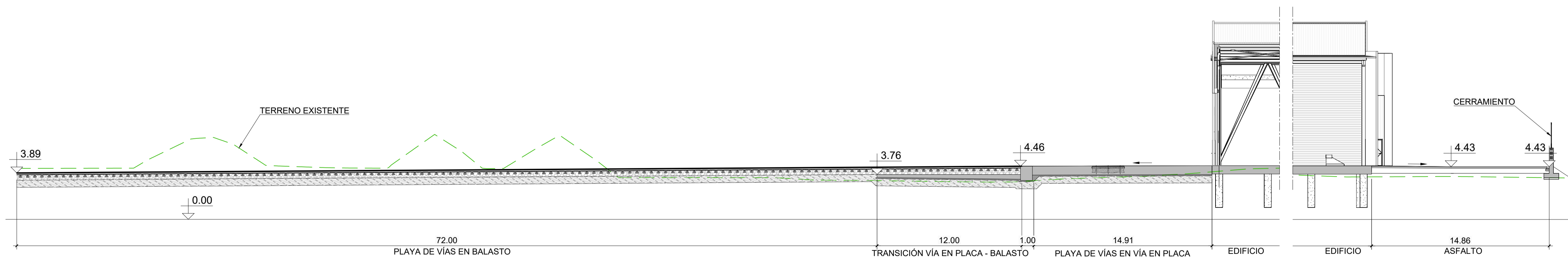
SECCIÓN C-C SCALE 1/200
