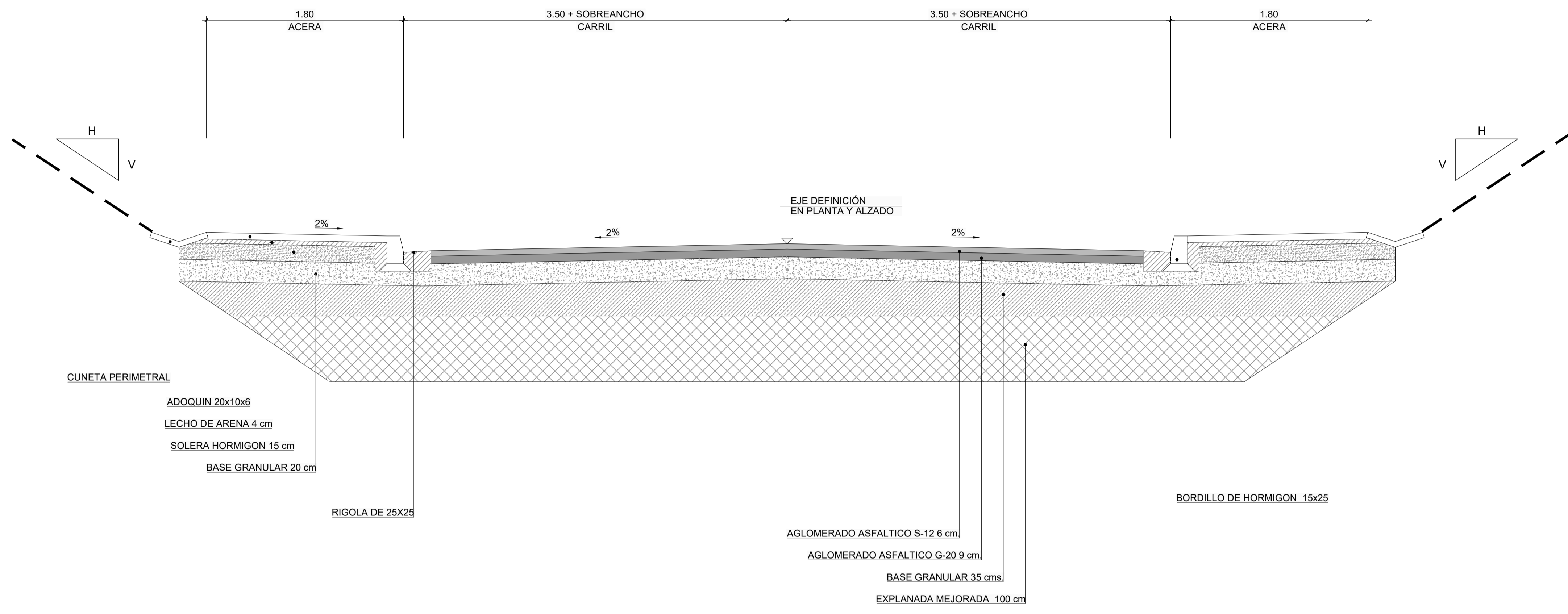
SECCIÓN TIPO VIAL DE ACCESO ESCALA 1/25
