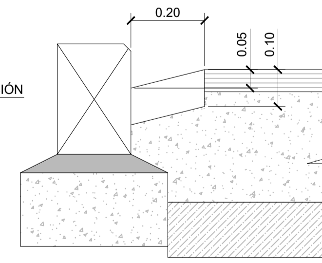
RIGOLA ESCALA 1:10
