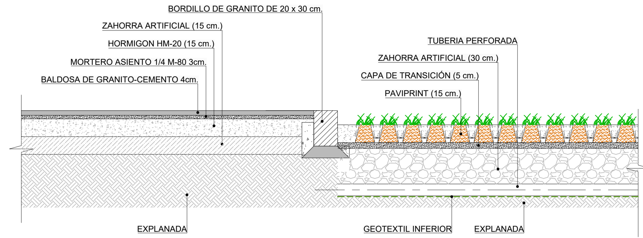
DETALLE 1 ESCALA 1:20
