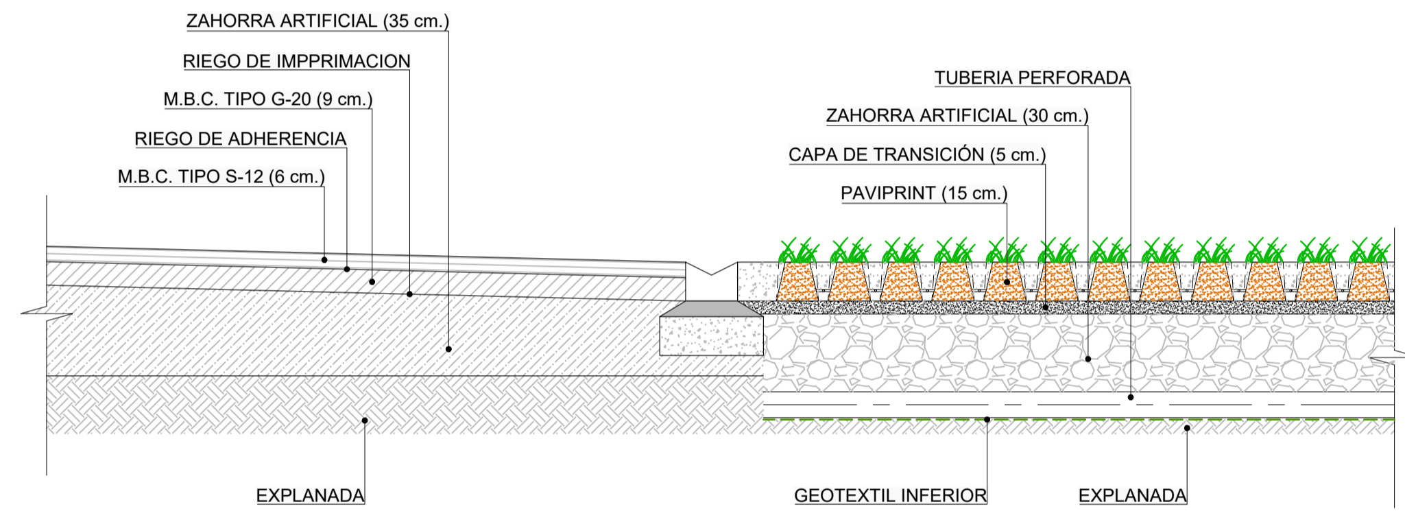
DETALLE 2 ESCALA 1:20
