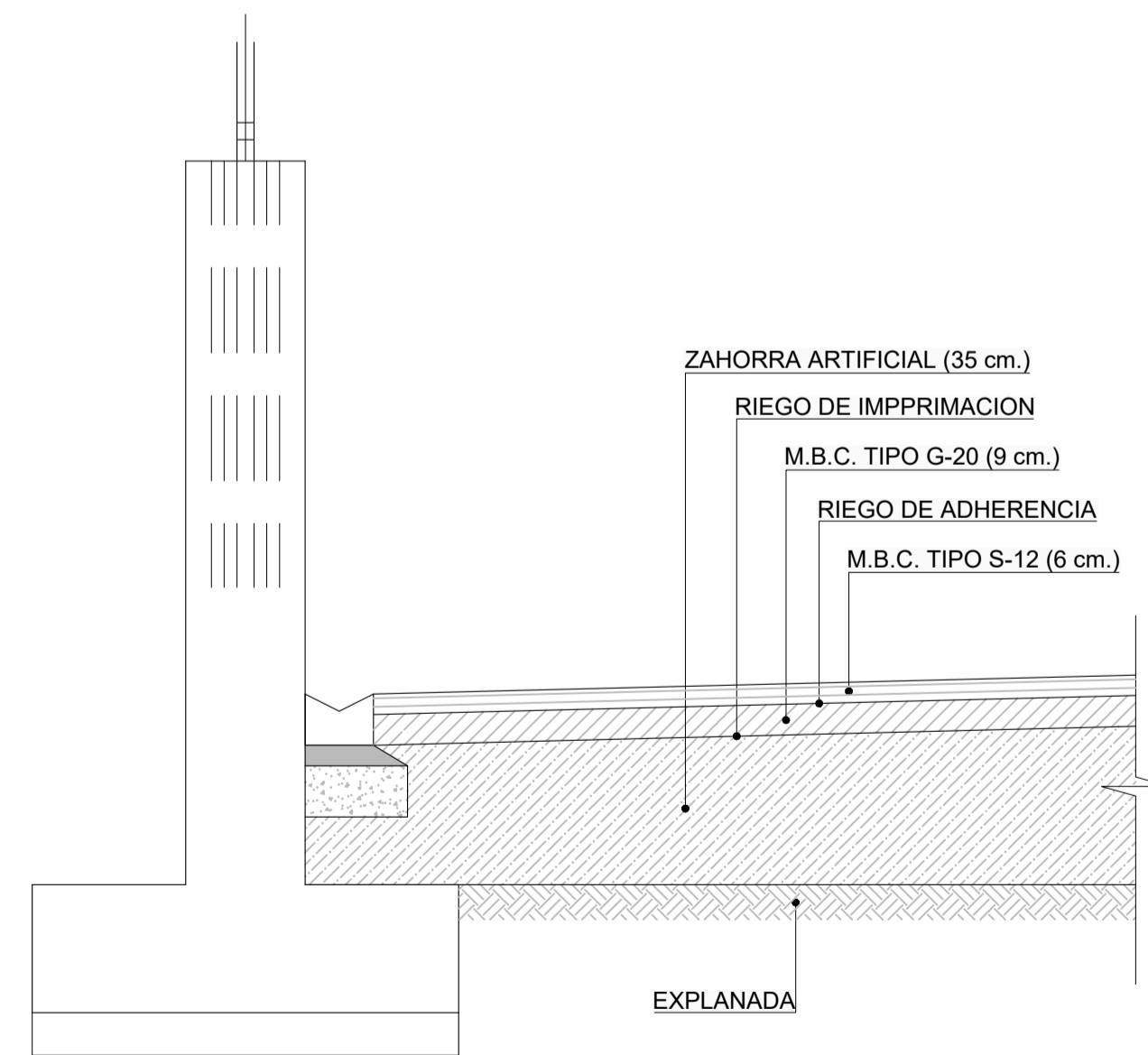
DETALLE 3 ESCALA 1:20
