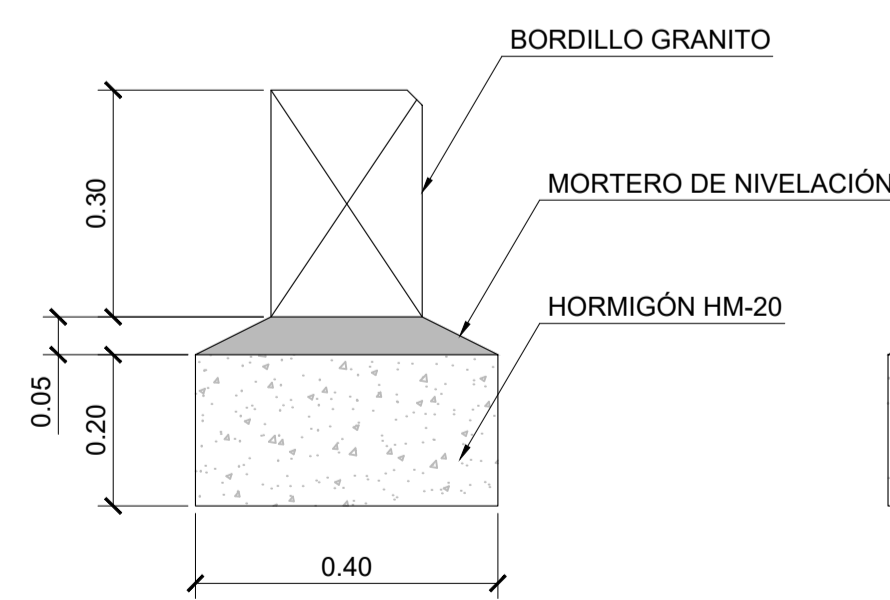
BORDILLO ESCALA 1:10
