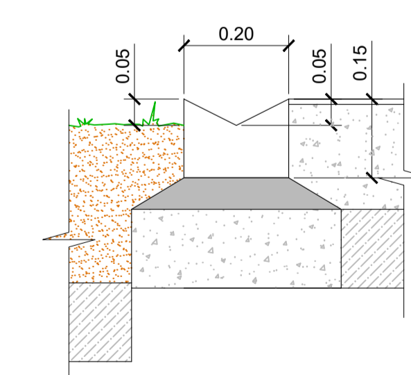
CAZ PREFABRICADO ESCALA 1:10
