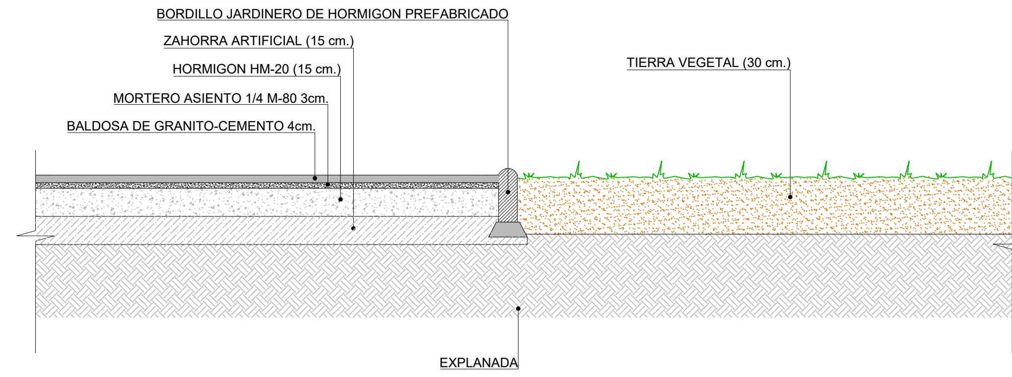
DETALLE 4 ESCALA 1:20
