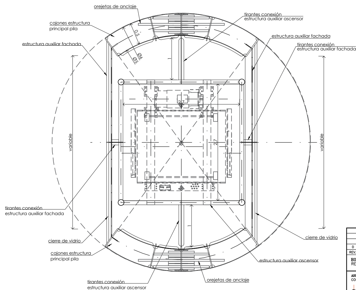
sección transversal zona baja pila escala: 1/25
