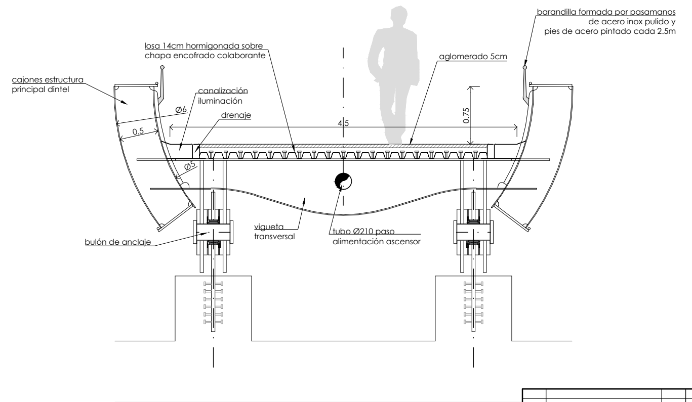
sección transversal desembarco San Roke escala: 1/25
