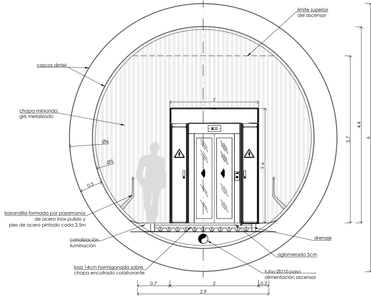
sección transversal desembarco ascensor escala: 1/25
