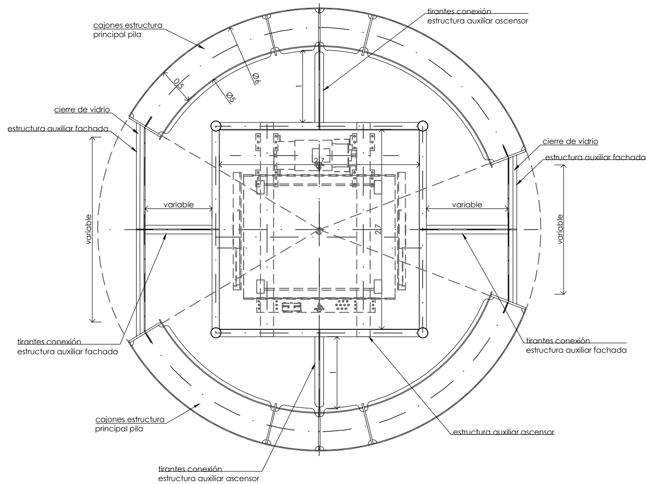
sección transversal zona superior pila escala: 1/25
