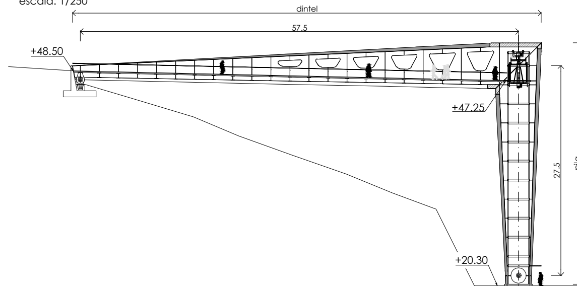
perfil longitudinal escala: 1/250
