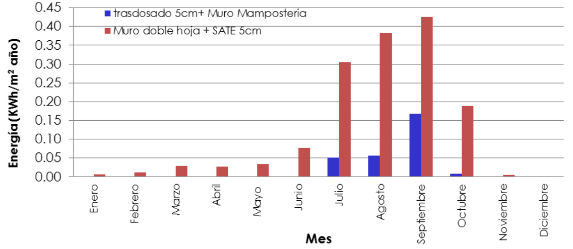
Figura 4.6. Ganancias Térmicas [kWh/m² mes] a lo largo del año en los dos cerramientos rehabilitados estudiados
