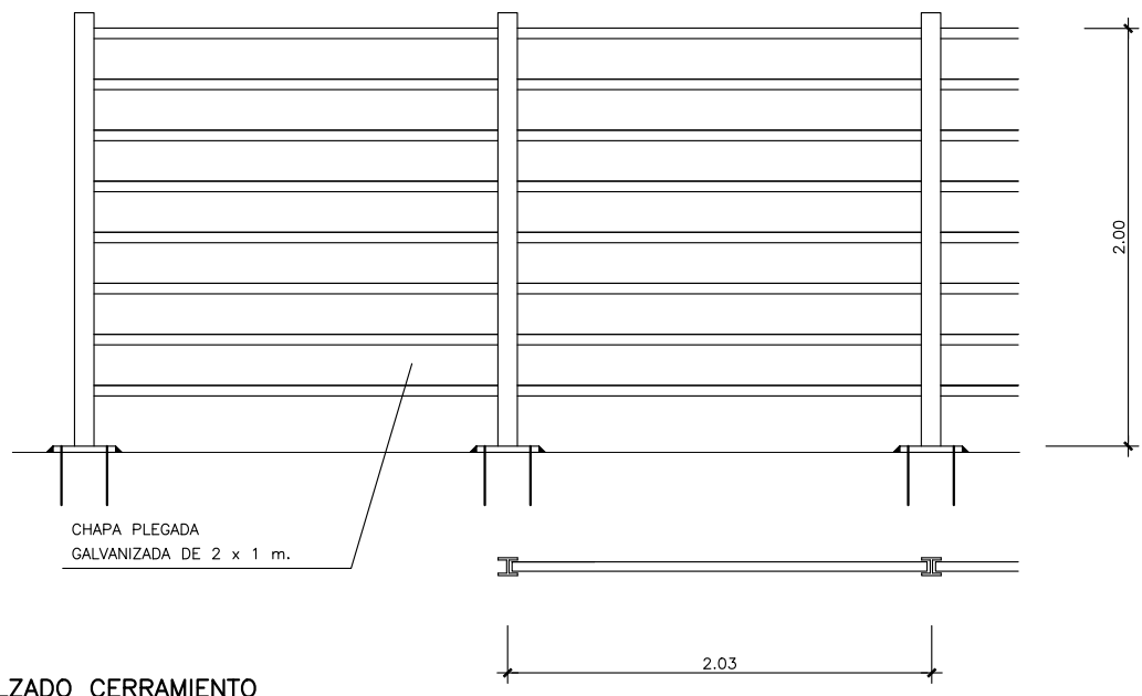
ALZADO CERRAMIENTO ESCALA 1:20
