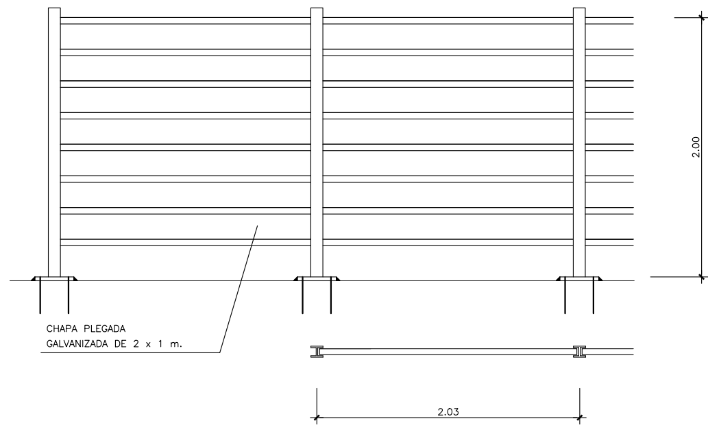
ALZADO CERRAMIENTO TRAFICO PEATONAL ESCALA 1:20
