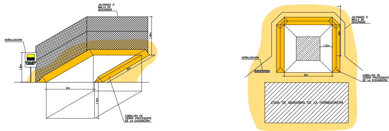
ZONA DE LIMPIEZA DE CANALETAS DE HORMIGONERAS
