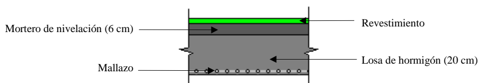
Fig. 3: Forjado de losa de hormigón de 20 cm
