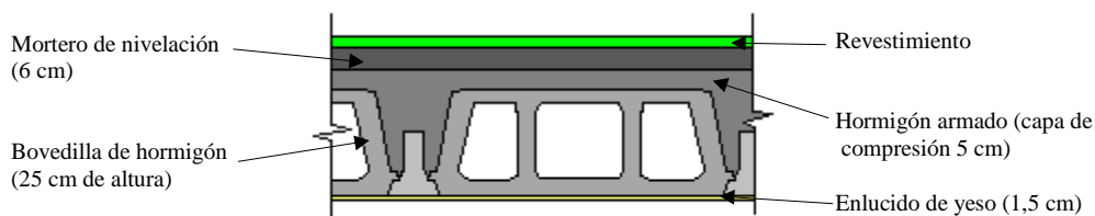
Fig. 1: Forjado de bovedillas de hormigón 25+5
