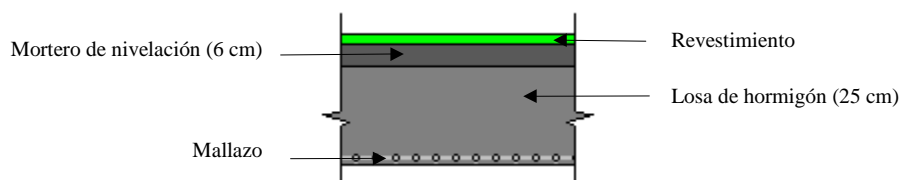
Fig. 4: Forjado de losa de hormigón de 25 cm
