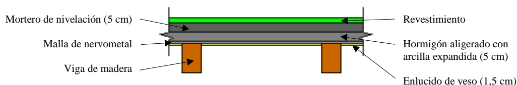
Fig. 5: Forjado ligero
