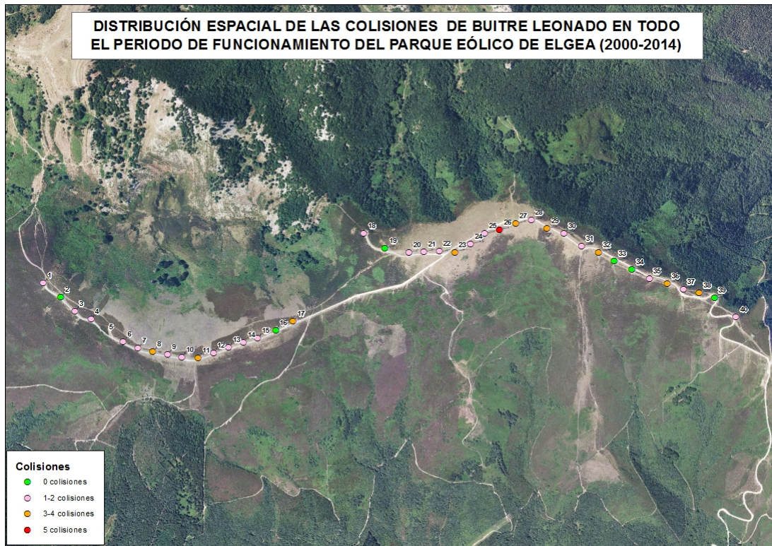
Figura 6: Distribución espacial de las colisiones de Buitre leonado en todo el periodo de funcionamiento del Parque Eólico de Elgea (2000-2014).
