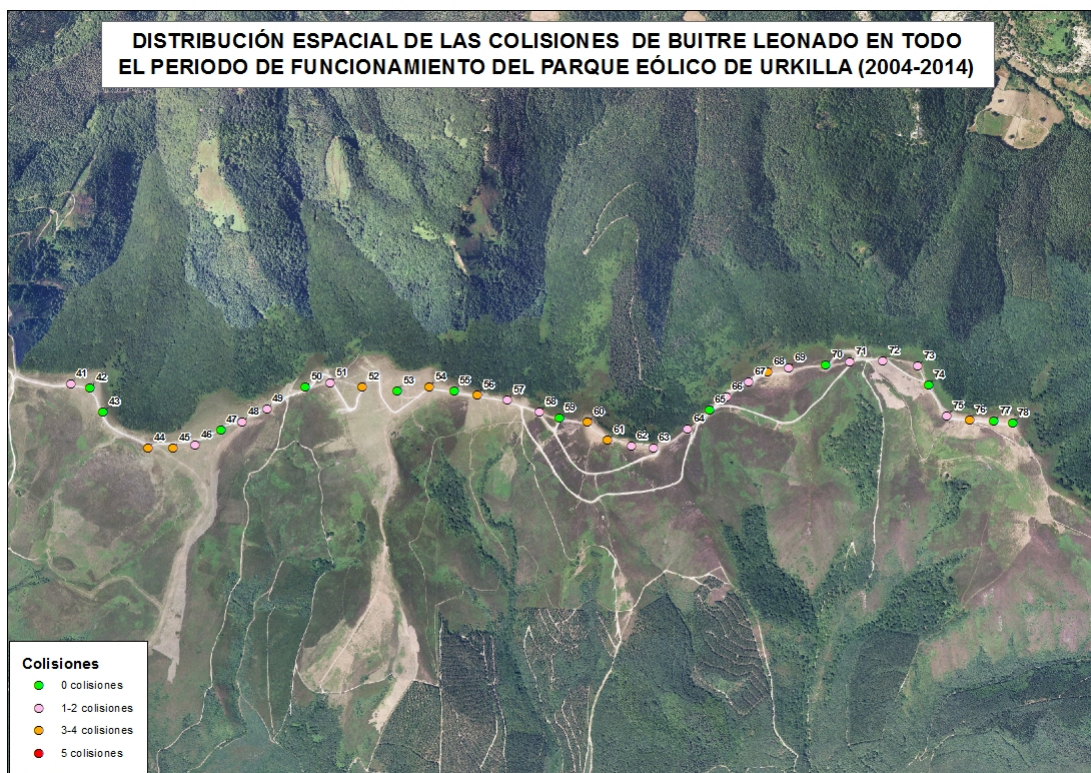
Figura 7: Distribución espacial de las colisiones de Buitre leonado en todo el periodo de funcionamiento del Parque Eólico de Urkilla (2004-2014).
