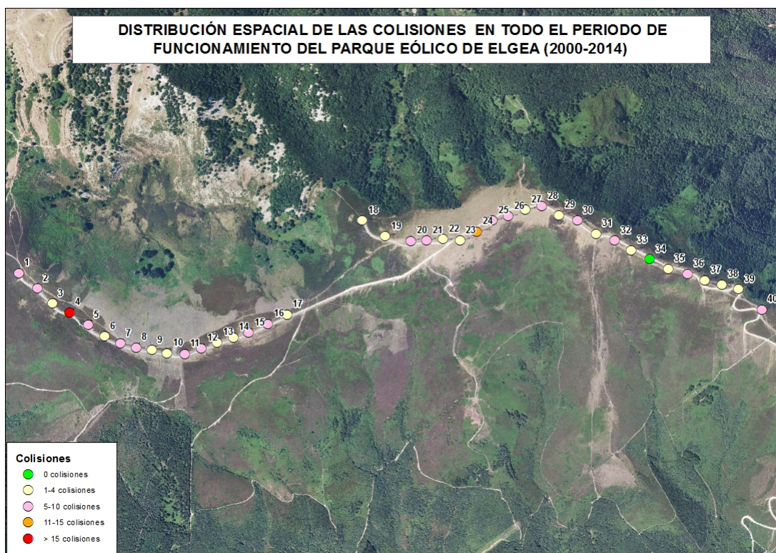
Figura 4: Distribución espacial de las colisiones en todo el periodo de funcionamiento del Parque Eólico de Elgea (2000-2014).
